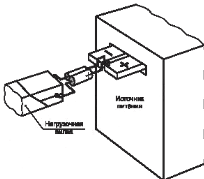
Рисунок А.2 — Схема для испытания дифференциальным измерением
