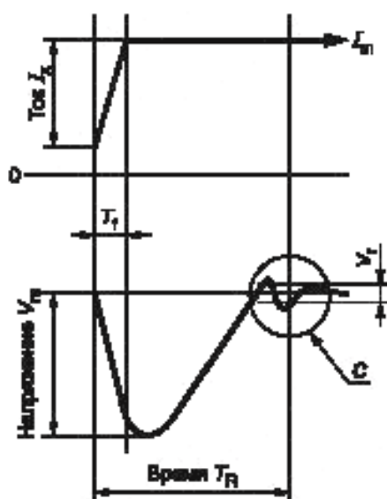
Рисунок 1 — Характеристика переходного процесса при активной нагрузке
