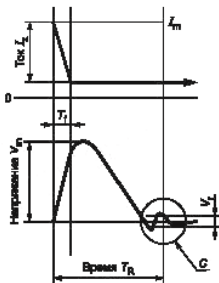
Рисунок 2 — Характеристика переходного процесса без активной нагрузки
