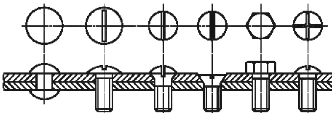
Рисунок А.7 — Пищевая зона. Крепеж, легко поддающийся очистке
