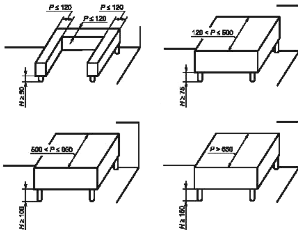
Рисунок А.8 — Подставки для печей хлебопекарных ротационных
