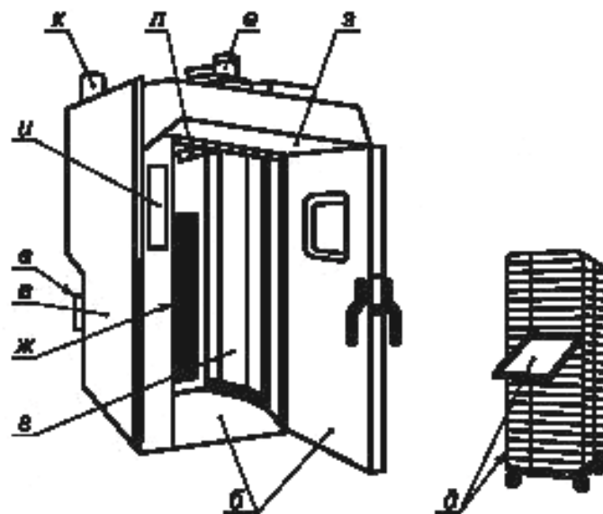
Рисунок 1 — Основные компоненты печи хлебопекарной ротационной
