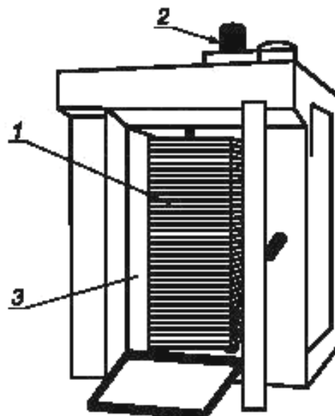
Рисунок 2 — Опасные зоны печи хлебопекарной ротационной
