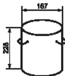
Рисунок 2 — Измерительный контейнер (малый)
