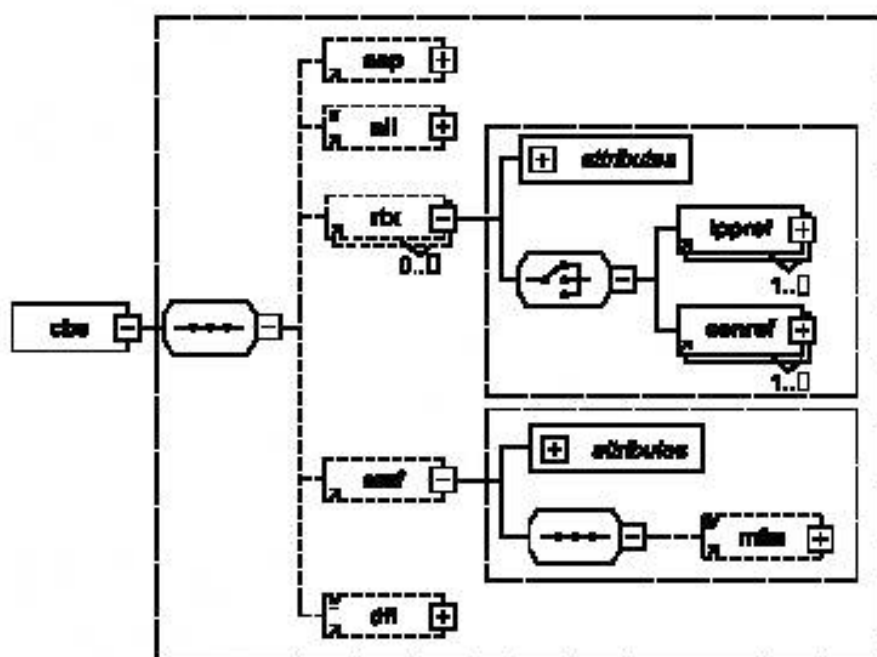
Рисунок 8 — Схема данных элемента CBS
