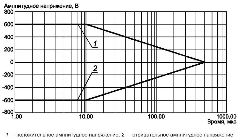
Рисунок 18 — Огибающие импульсов напряжения для приемников постоянного и переменного токов
