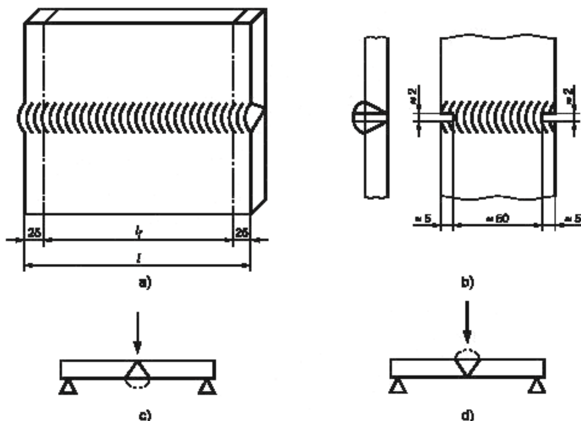
а) резка на четное количество образцов; б) участок, подлежащий испытанию; в) испытание на изгиб с лицевой стороны; г) испытание на изгиб со стороны корня шва
