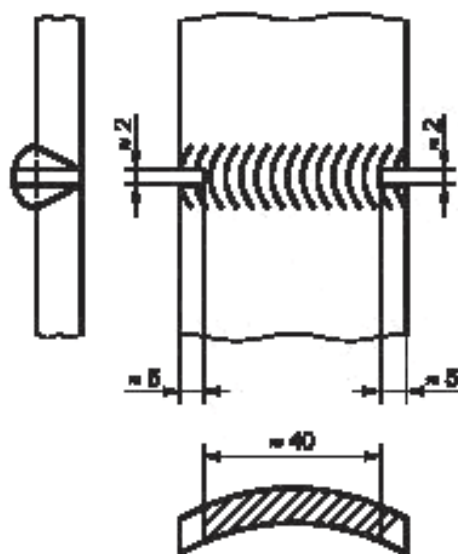
с) Участок, подлежащий испытанию
