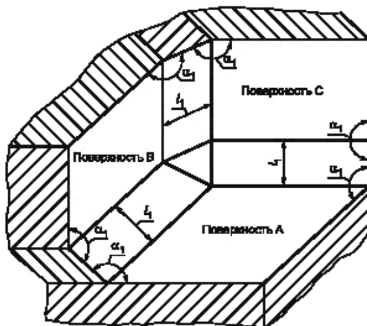
Рисунок A.4 — Пищевая зона
