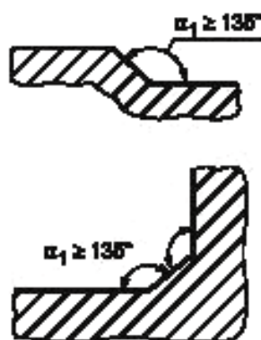
Рисунок A.3 — Пищевая зона
