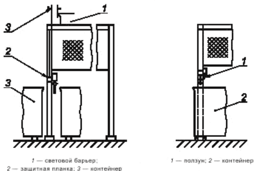
Рисунок 11 — Устройство блокировки положения контейнера
