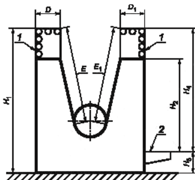
1 — механическая защитная планка; 2 — заблокированная площадка обслуживания
