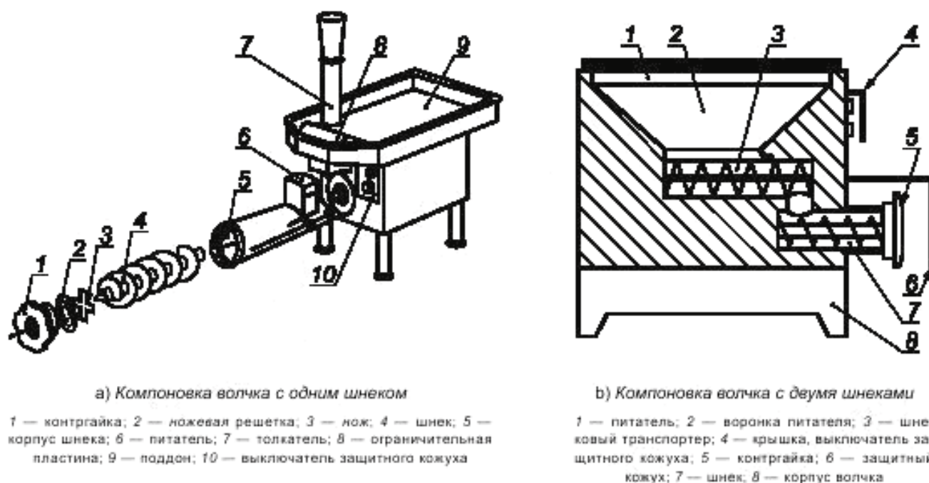
Рисунок 1 — Волчки для измельчения мяса и рыбы
