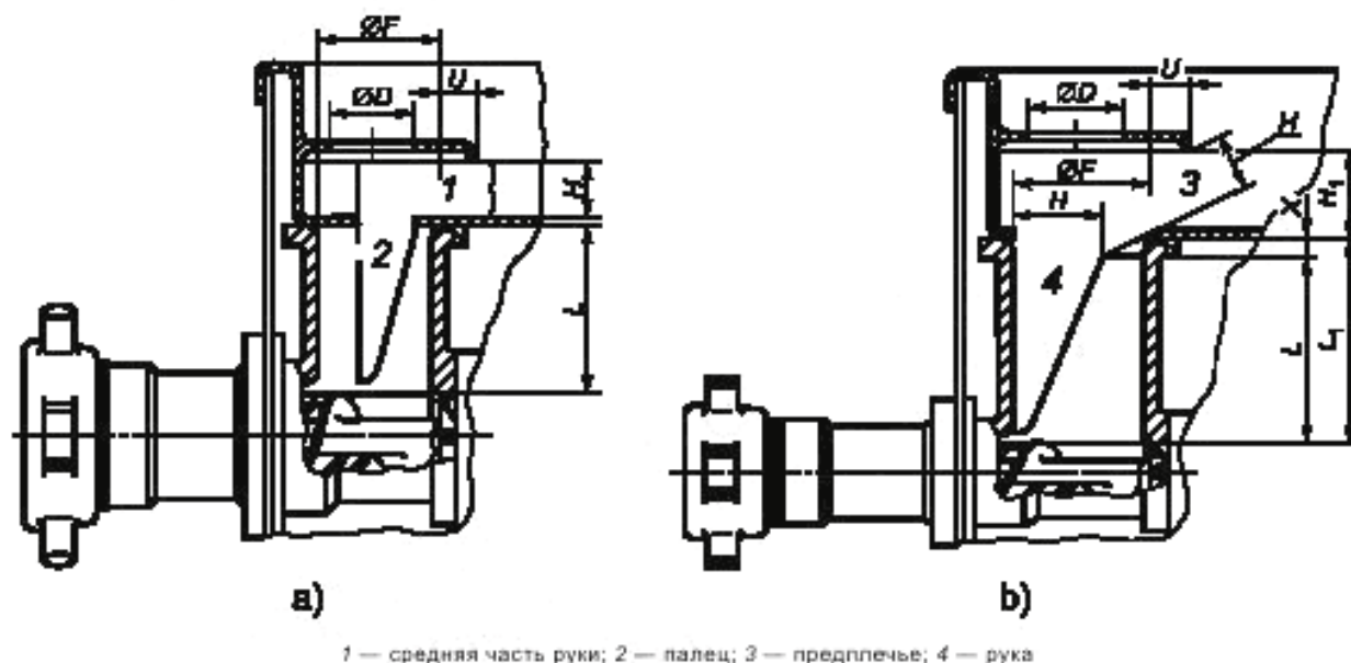
Рисунок 6 — Питатель с ограничительной пластиной. Безопасные размеры
