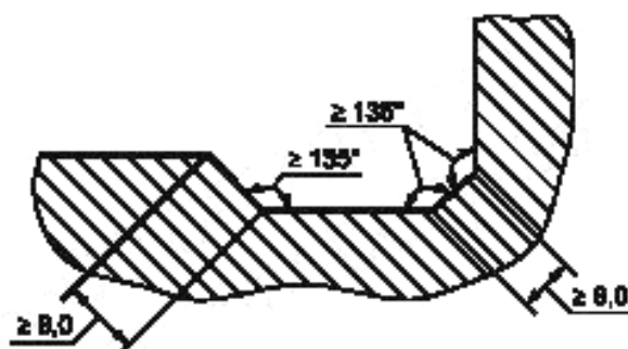
Рисунок А.3 — Углы в пищевой зоне
