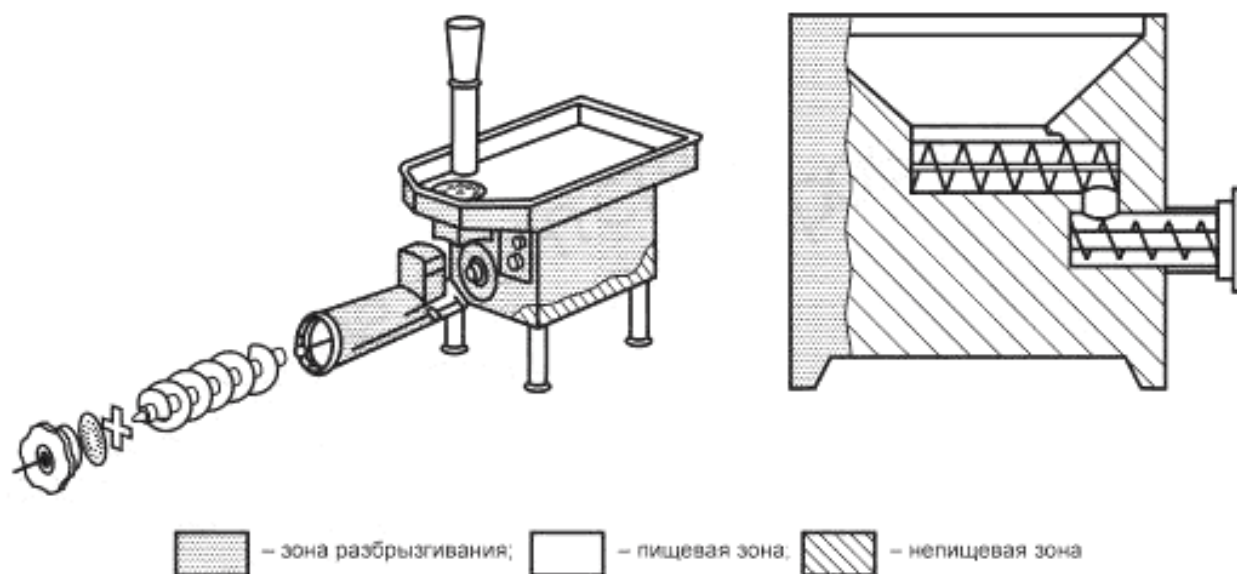
Рисунок 13 — Гигиенические зоны волчка
