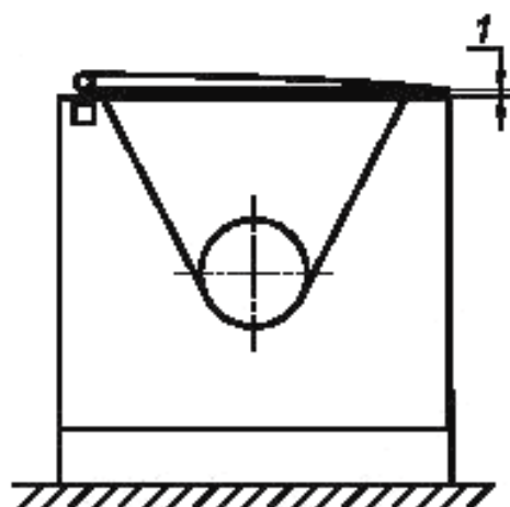
1 — расстояние открывания заблокированной крышки
