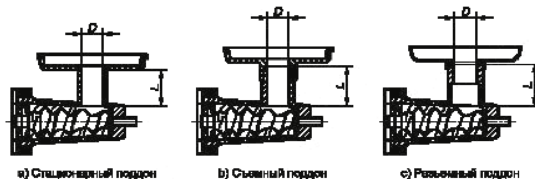
Рисунок 5 — Питатель без ограничительной пластины. Безопасные размеры
