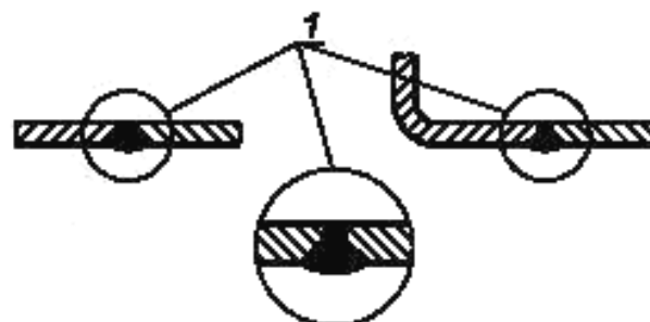
Рисунок А.1 — Гладкие поверхности. Пищевая зона
