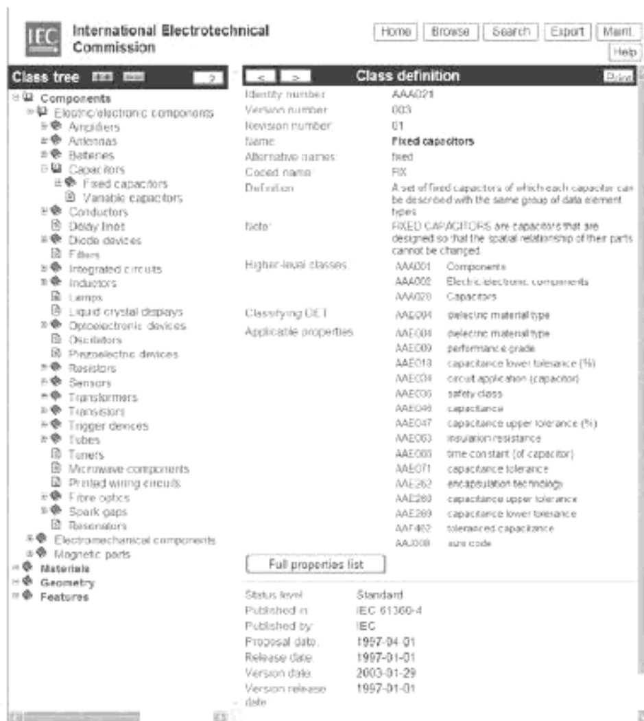
Рисунок 6 — Примеры классификации типов элементов данных (DET)
