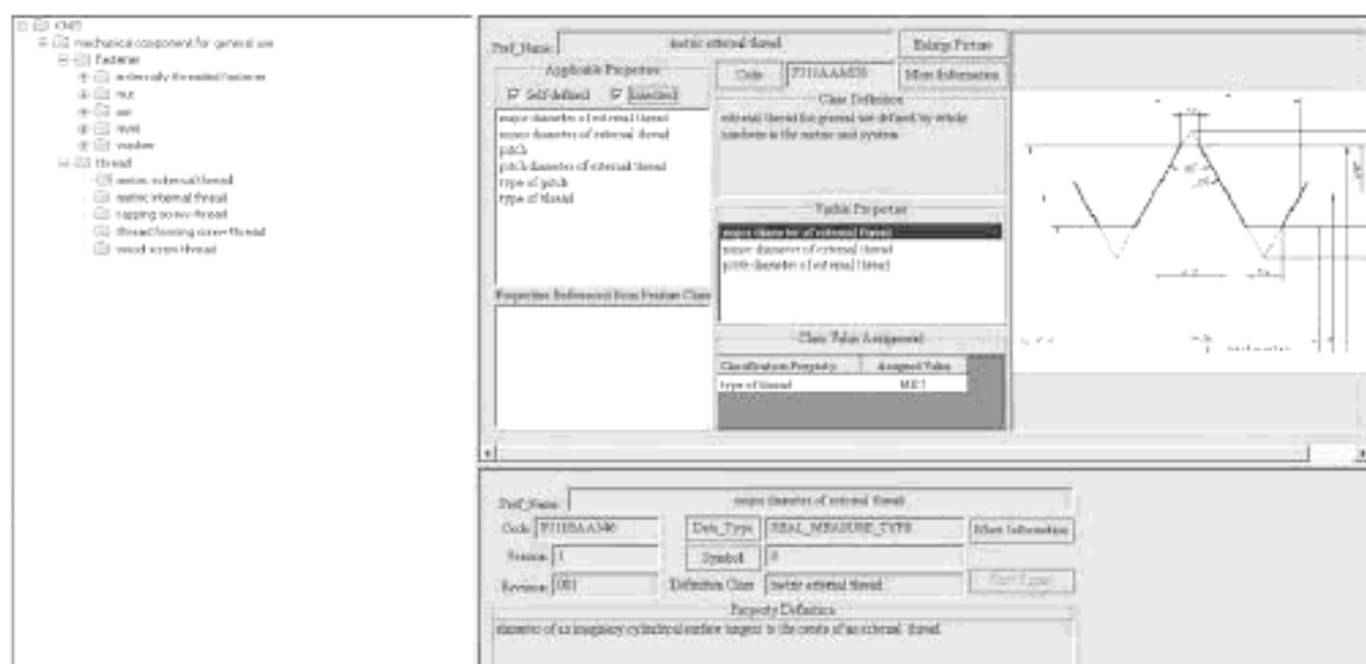
Рисунок 4 — Характеристический класс резьбы по ISO 13584-511
