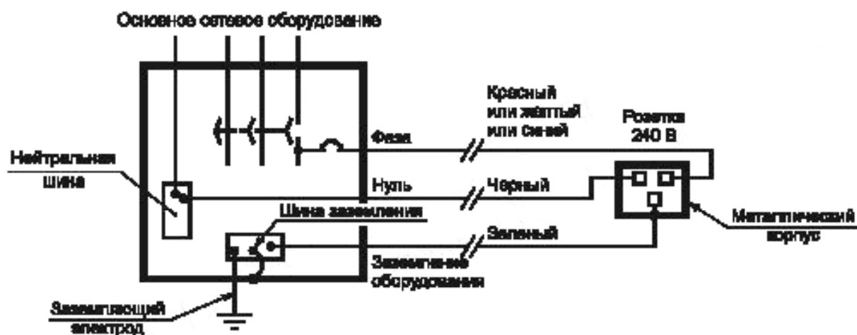
Рисунок 4б — Пример Малазийской энергосистемы
