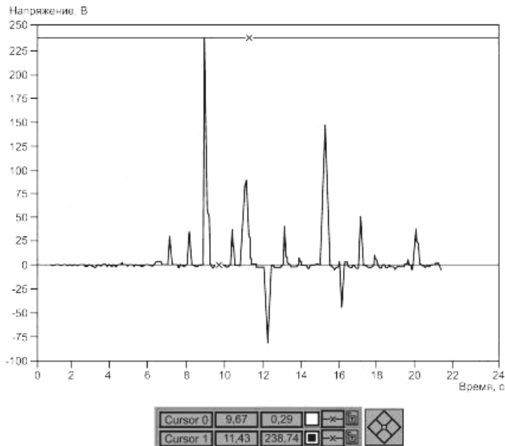
Рисунок В — Напряжение на сотруднике, идущем по заземленному проводящему полу с двумя надетыми ремешками заземления
