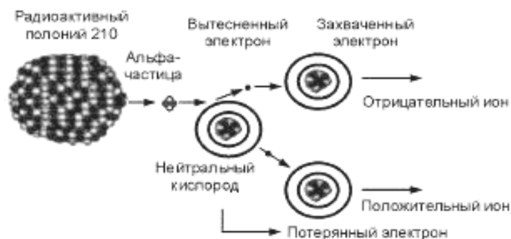
Рисунок 9 — Ионизация альфа-излучением
