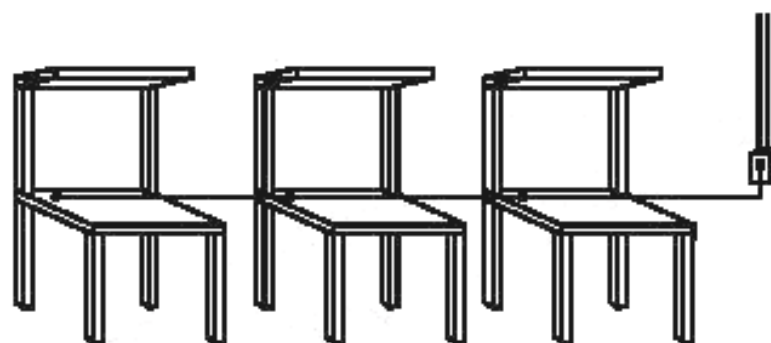
Рисунок 6 — Пример нерекомендуемого заземления последовательно соединенных столов
