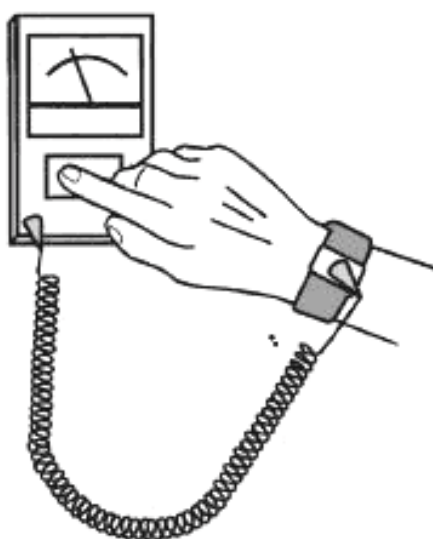
Рисунок А.1 — Испытание антистатического браслета
