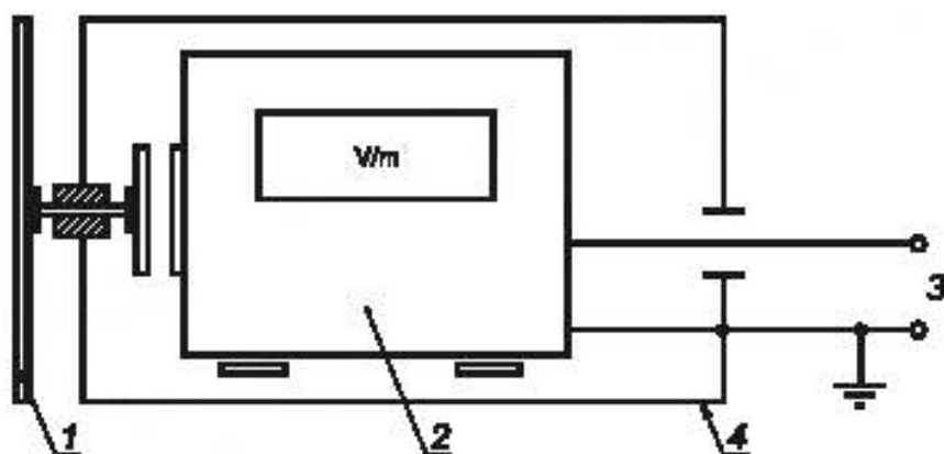
1 — изолированный электрод; 2 — измеритель поля; 3 — внешний выход; 4 — экран
