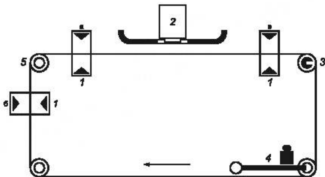
а — оценка эффективности нейтрализации; б — наблюдение заряда свободного ролика; в — вторичный прикладываемый заряд; 1 — нейтрлизатор; 2 — измеритель поля; 3 — ролик с приводом; 4 — подвижная ось с нагрузкой на ленту; 5 — свободно вращающиеся ролики
