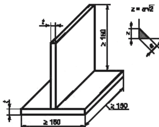
\alpha — номинальная толщина шва, мм; (0,5t \leq \alpha \leq 0,7t) t — толщина материала контрольного сварного соединения, мм; z — величина катета углового шва (мм);
