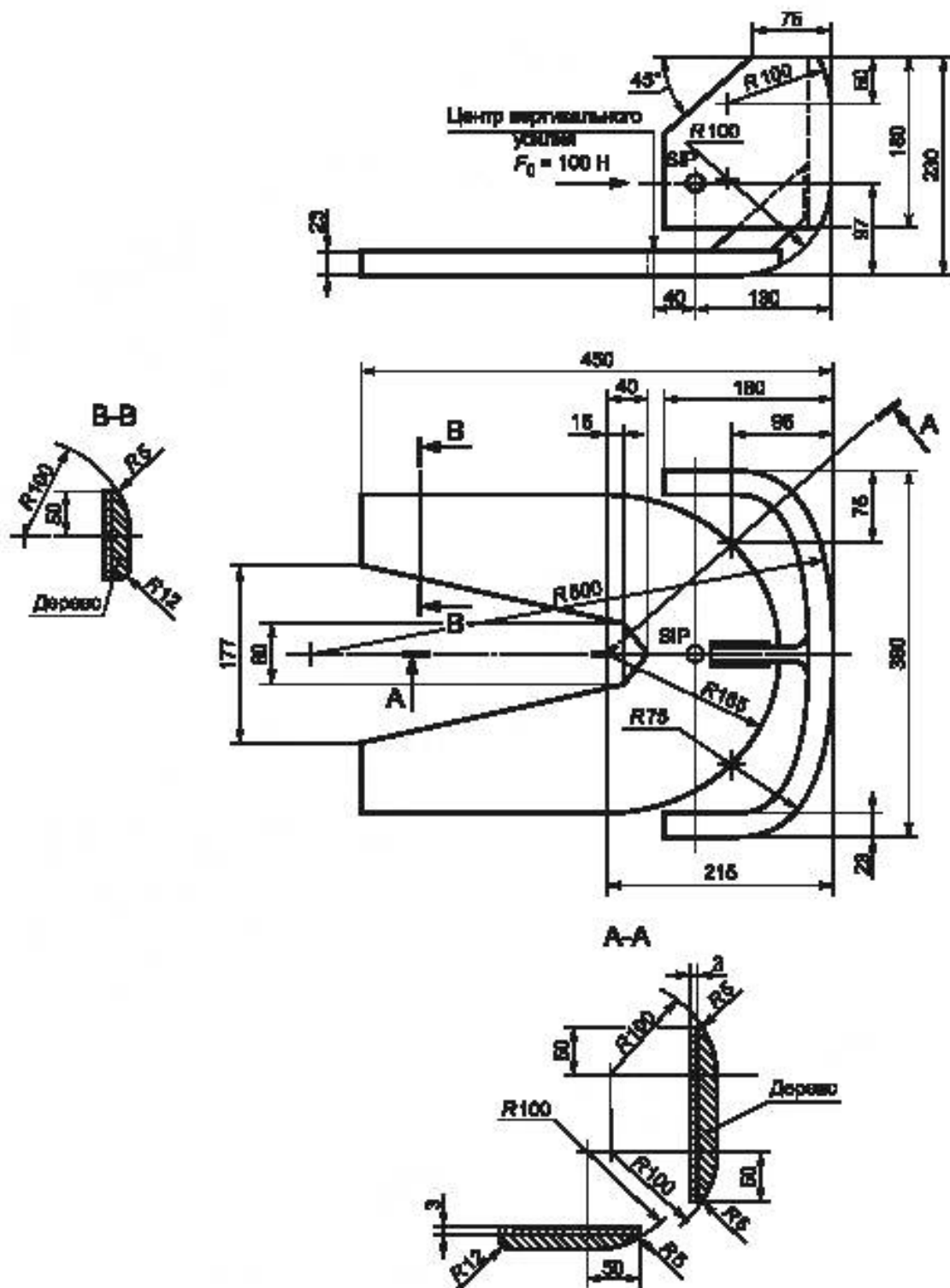
Рисунок 1 — Устройство для определения контрольной точки сиденья
