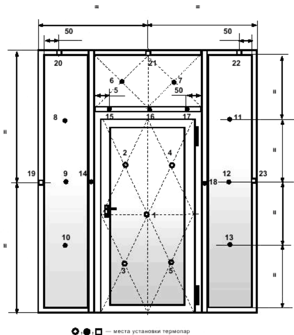
Рисунок А.9 — Схема установки термодатчиков на необогреваемых поверхностях перегородки и вмонтированного в нее однопольного дверного блока со светопропускающими элементами
