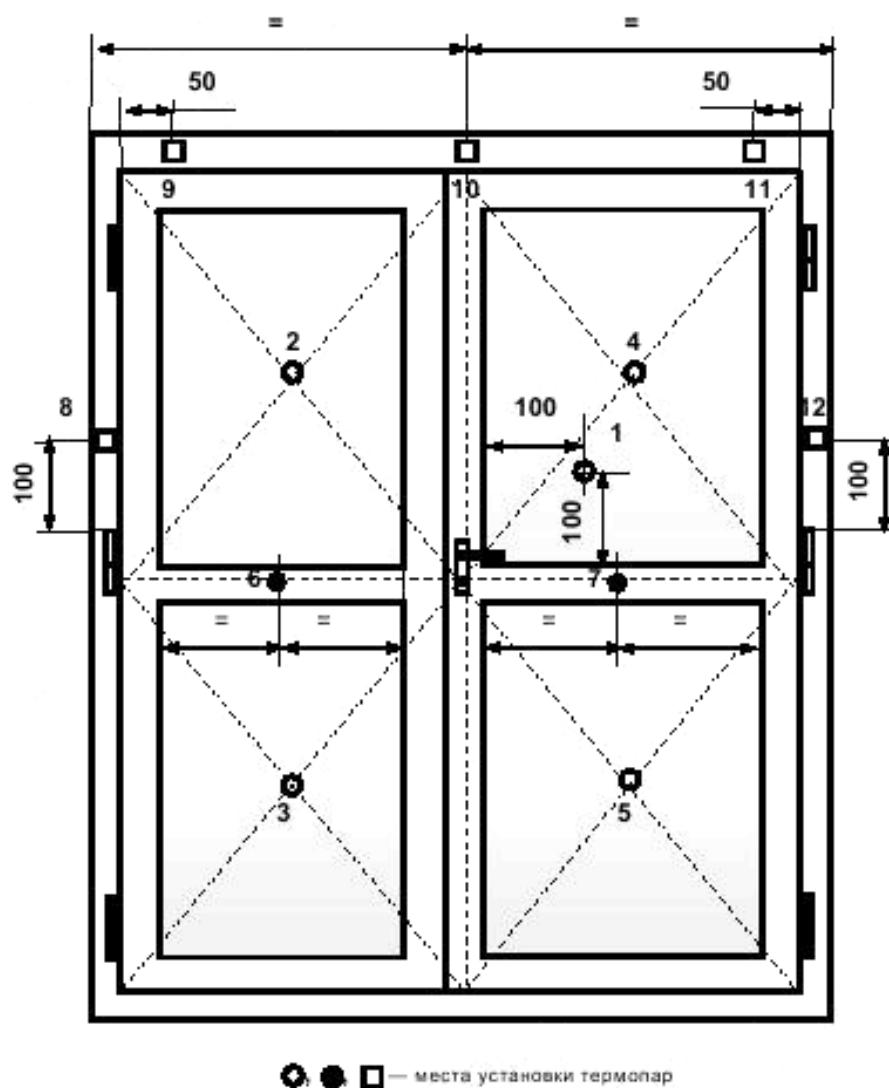
Рисунок А.7 — Схема установки термодпар на необогреваемой поверхности двухпольного дверного блока
