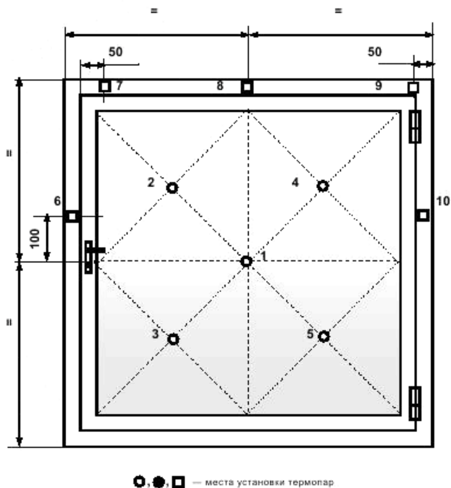
Рисунок А.12 — Схема установки термодпар на необогреваемой поверхности люка
