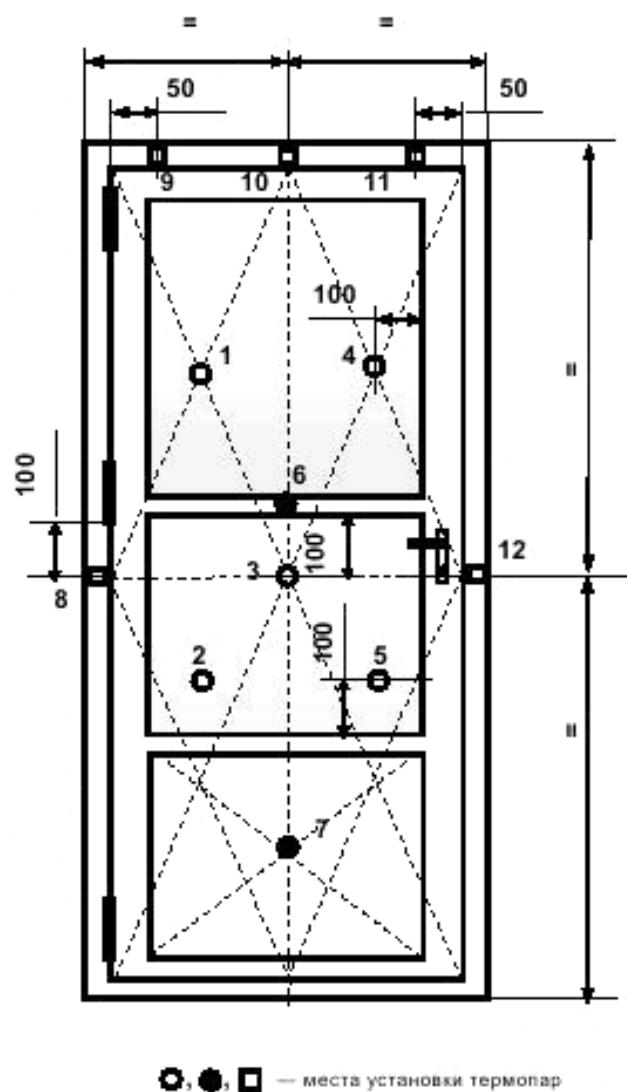
Рисунок А.5 — Схема установки термопар на необогреваемой поверхности однопольного дверного блока
