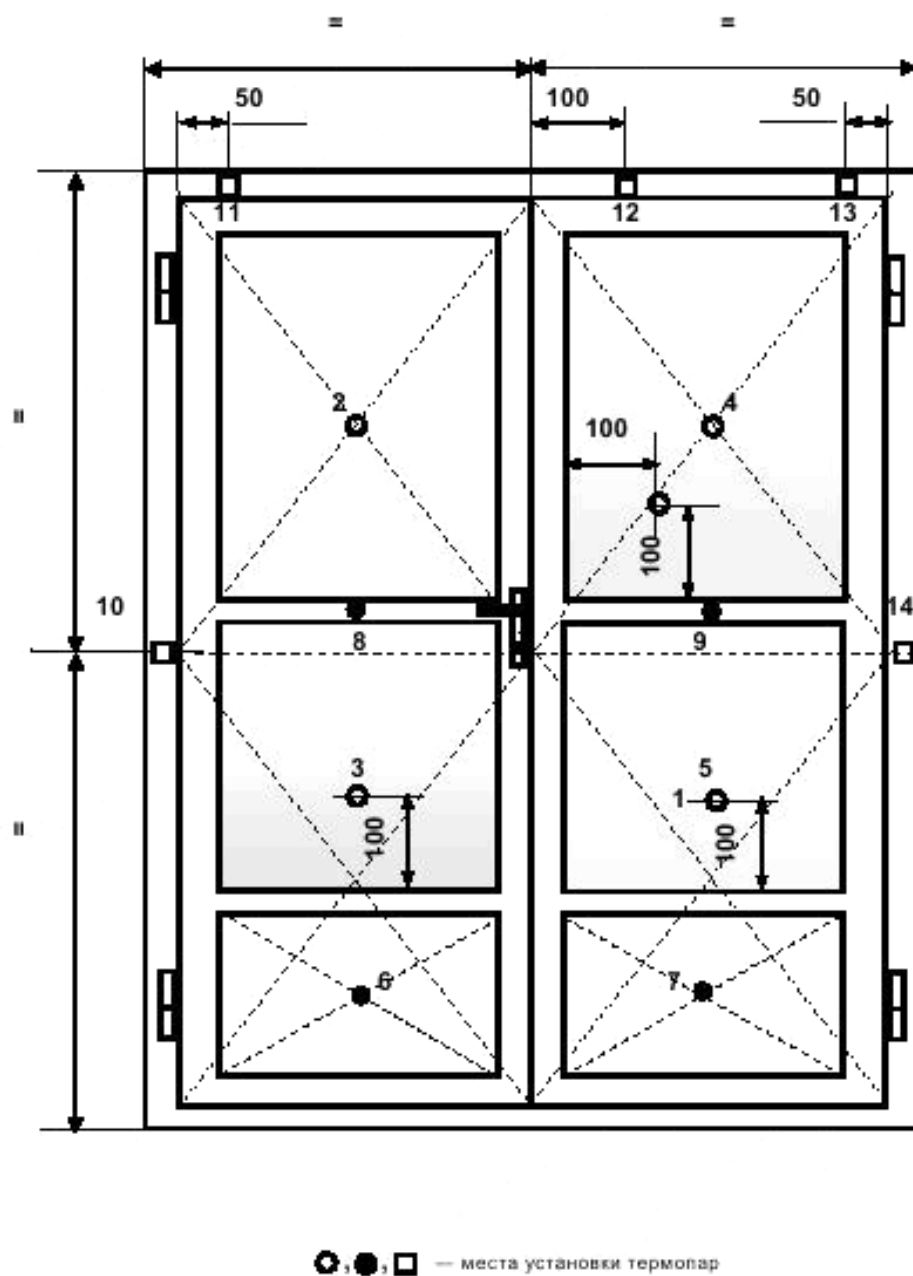
Рисунок А.6 — Схема установки термопар на необогреваемой поверхности двухпольного дверного блока
