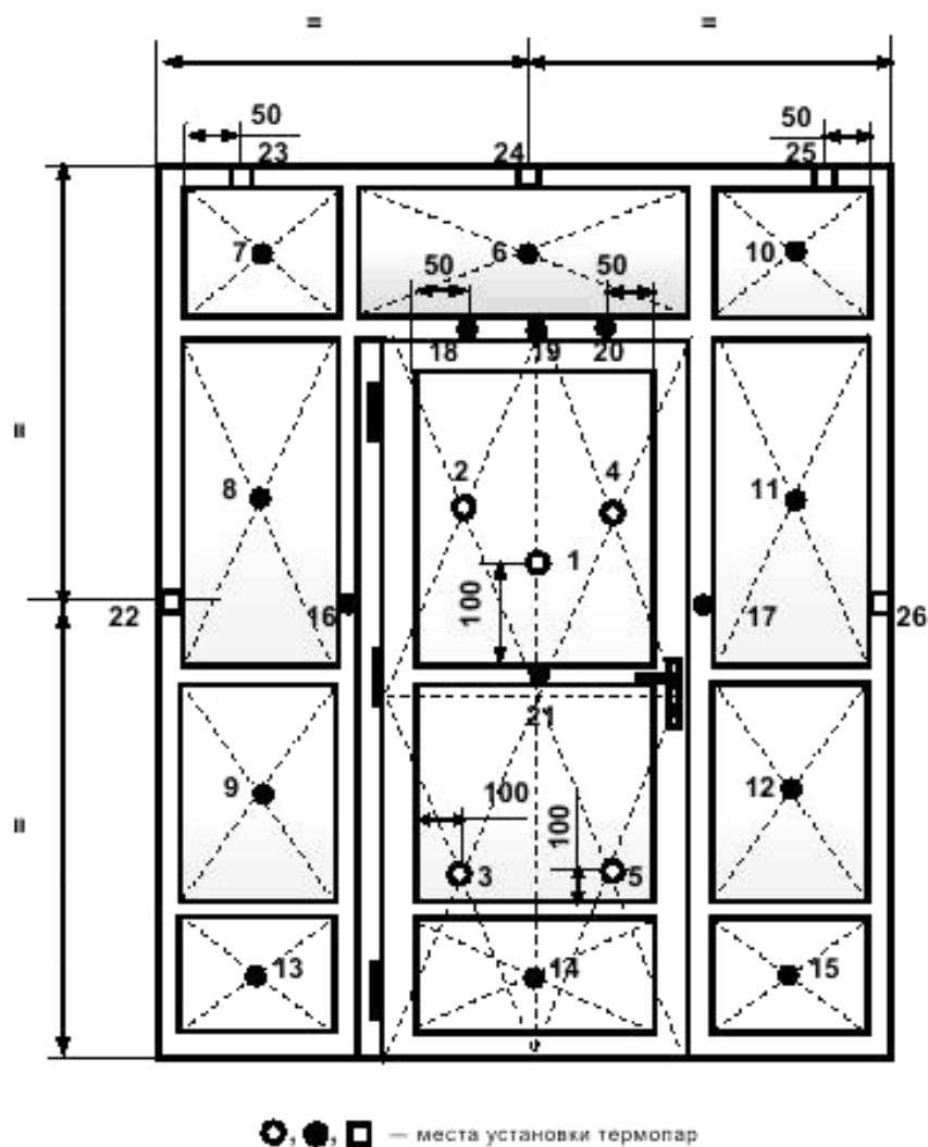
Рисунок А.10 — Схема установки термодатчиков на необогреваемых поверхностях перегородки и вмонтированного в нее однопольного дверного блока со светопропускающими и глухими элементами
