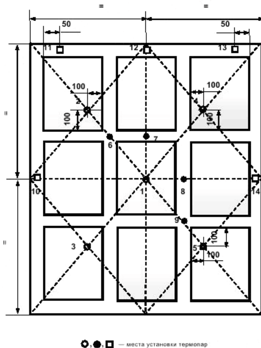
Рисунок А.2 — Схема установки термодатчиков на неотапливаемой поверхности перегородки
