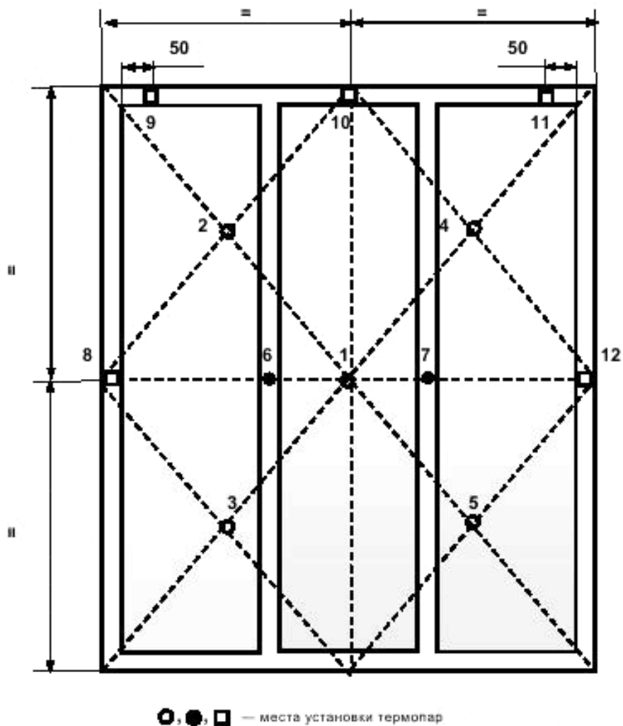
Рисунок А.1 — Схема установки термодатчиков на необогреваемой поверхности перегородки или перекрытия
