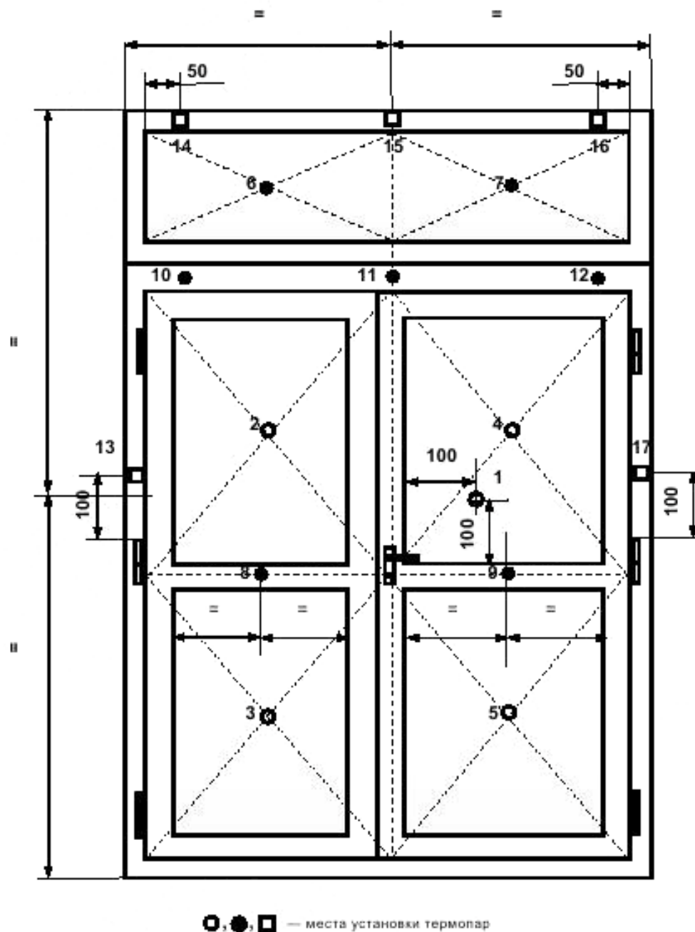
Рисунок А.8 — Схема установки термодатчиков на необогреваемой поверхности двухпольного дверного блока с фрамугой
