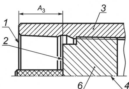
в — контроль трубной резьбы трапецеидального профиля гладким калибром-пробкой
