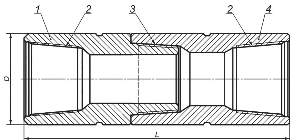
1 — ниппель; 2 — трубная резьба треугольного профиля; 3 — замковая резьба; 4 — муфта; D — наружный диаметр замка; L — длина замка
