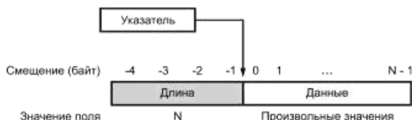
Рисунок 5 — Структура блока данных в памяти
