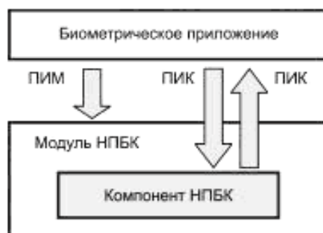
Рисунок 3 — Модель взаимодействия ПИМ/ПИК НПБК
