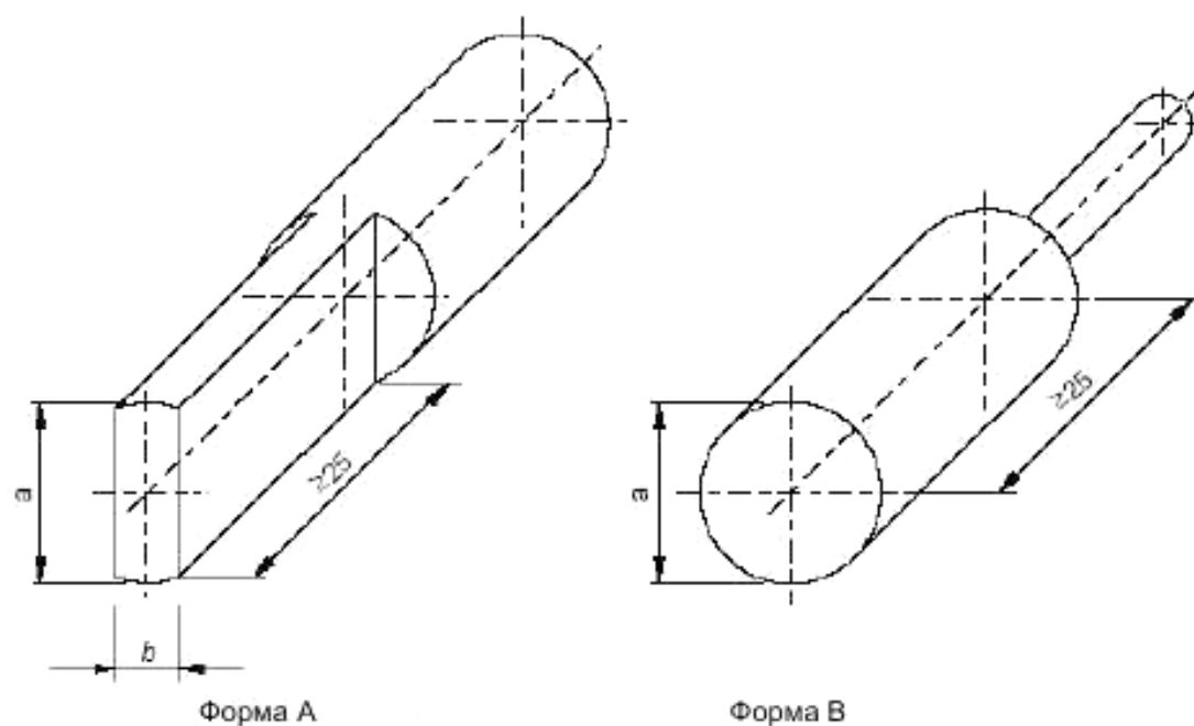
Рисунок 2 – Калибры
