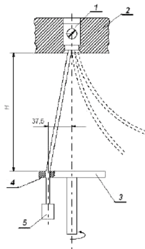
Рисунок 1 – Испытательная установка (9.4)
