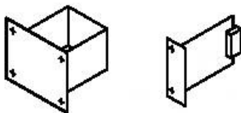
Рисунок 4 — Примеры исполнения вставного блока
