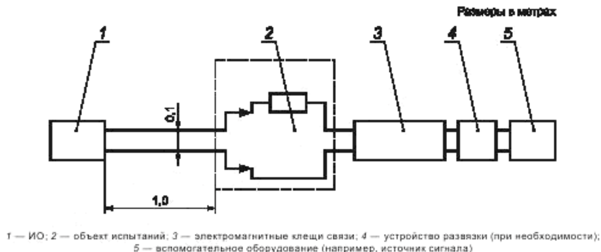
Рисунок 2 — Пример соединений при измерении напряжения
