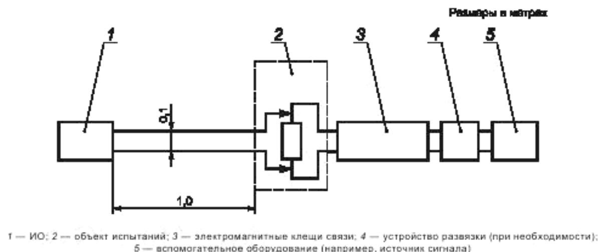
Рисунок 3 — Пример соединений при измерении тока
