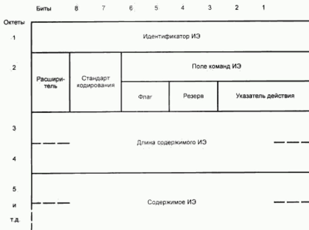
Рисунок 3 — Структура формата ИЭ
