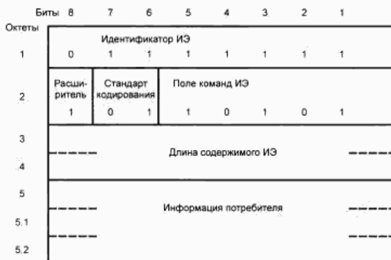
Рисунок 17 — Формат ИЭ «Информация потребитель—потребитель»
