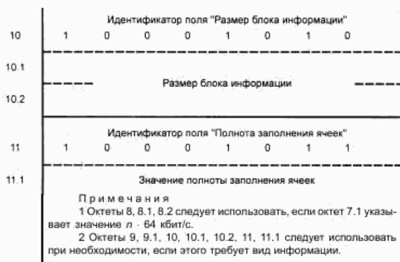
Рисунок 4 — Формат ИЭ «Параметры уровня адаптации» типа 1
