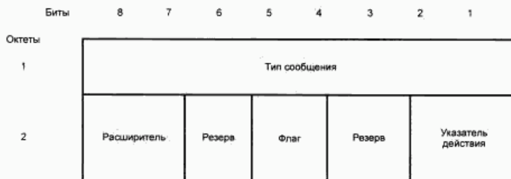
Рисунок 2 — Структура поля «Тип сообщения»
