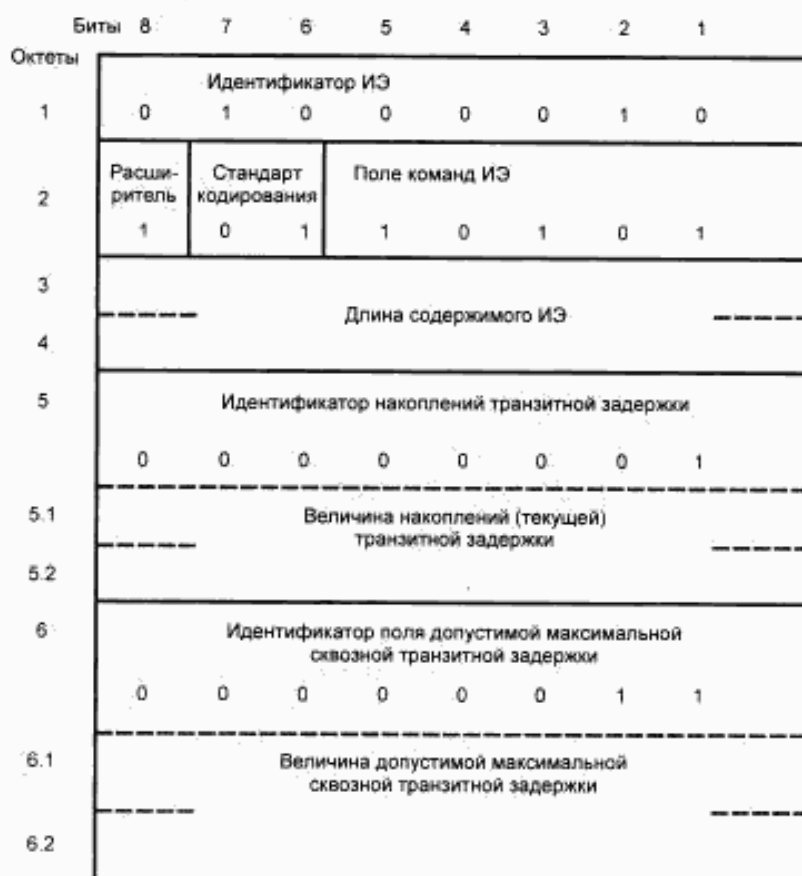
Рисунок 14 — Формат ИЭ «Сквозная транзитная задержка»
