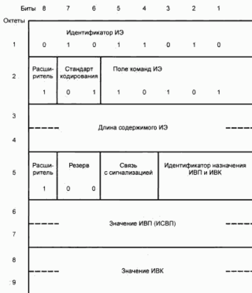
Рисунок 11 — Формат ИЭ «Идентификатор виртуального соединения»
