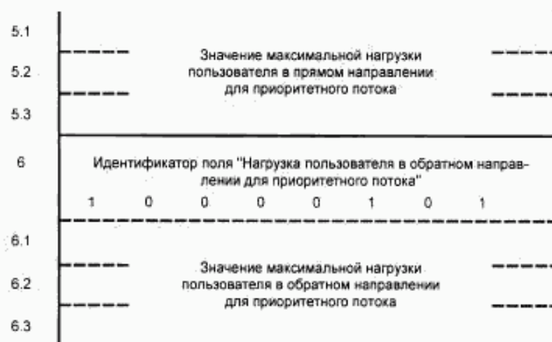
Рисунок 12 — Формат ИЭ «Идентификатор нагрузки пользователя»
