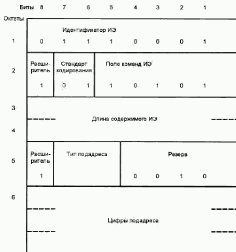
Рисунок 10 — Формат ИЭ «Субадрес вызываемой стороны»
