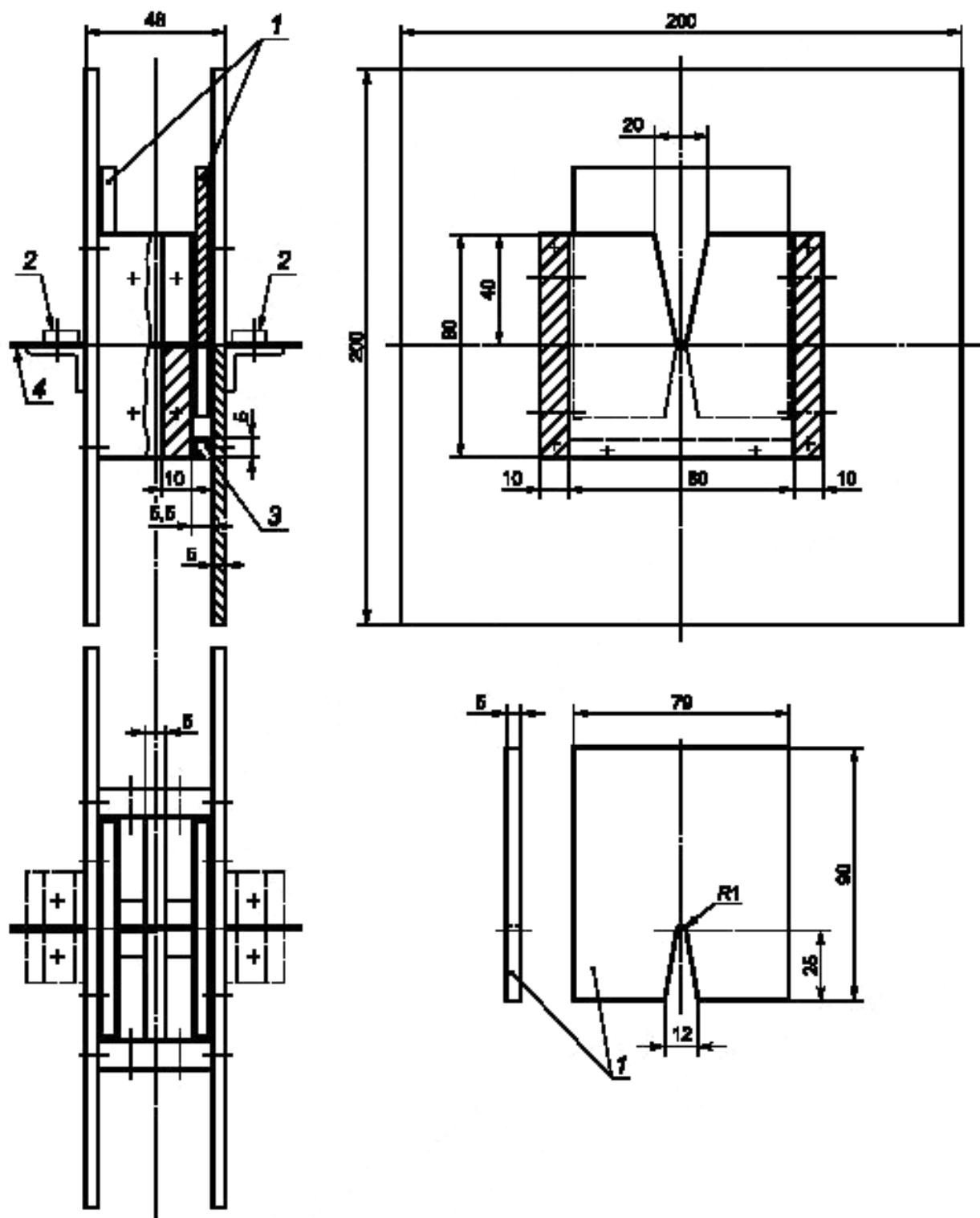
Рисунок 105 – Испытательная установка для проверки минимальных значений \hat{P}t и I_p , выдерживаемых выключателем-разъединителем
