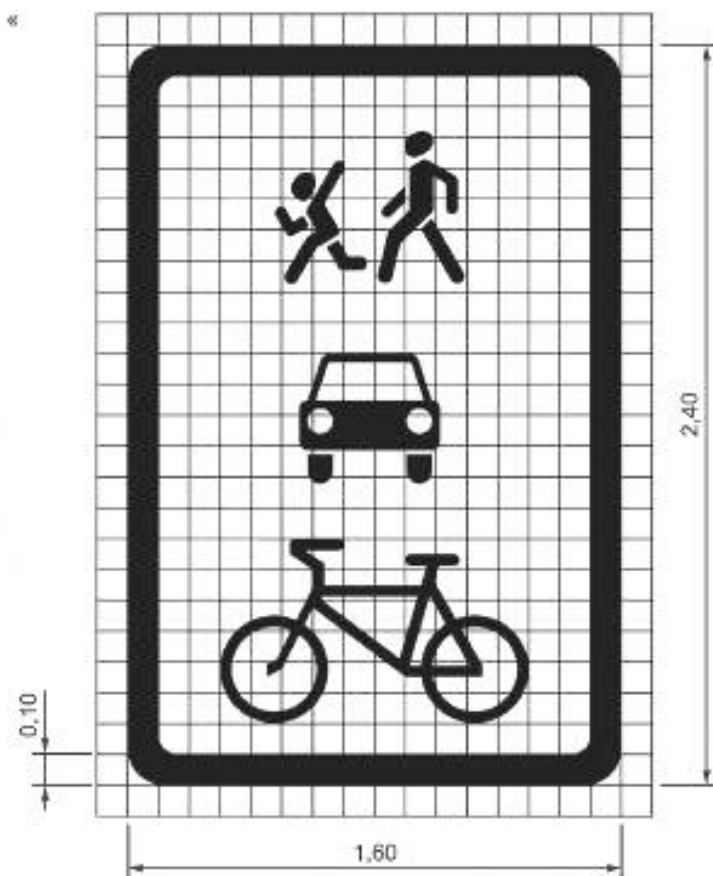
Рисунок Б.19 — Размеры разметки 1.24.6
