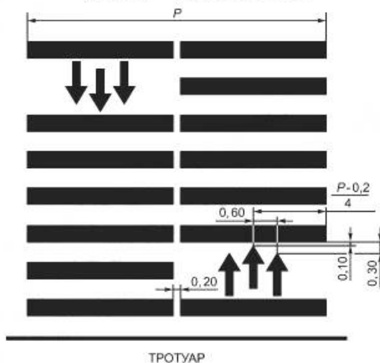
Рисунок Б.2 — Расположение стрел на разметке 1.14.2
