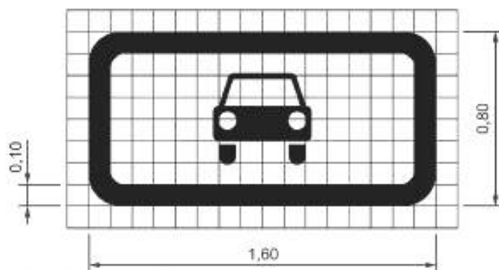
Рисунок Б.20 — Размеры разметки 1.24.7».
