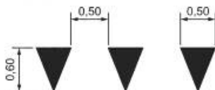
Рисунок Б.1 — Размеры разметки 1.13
