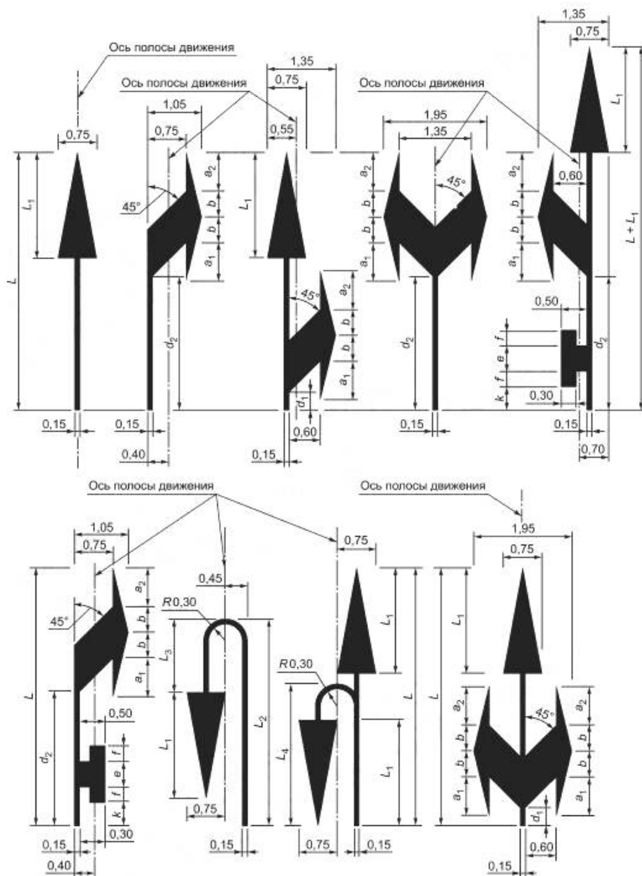
Рисунок Б.5 — Размеры стрел разметки типа 1.18
