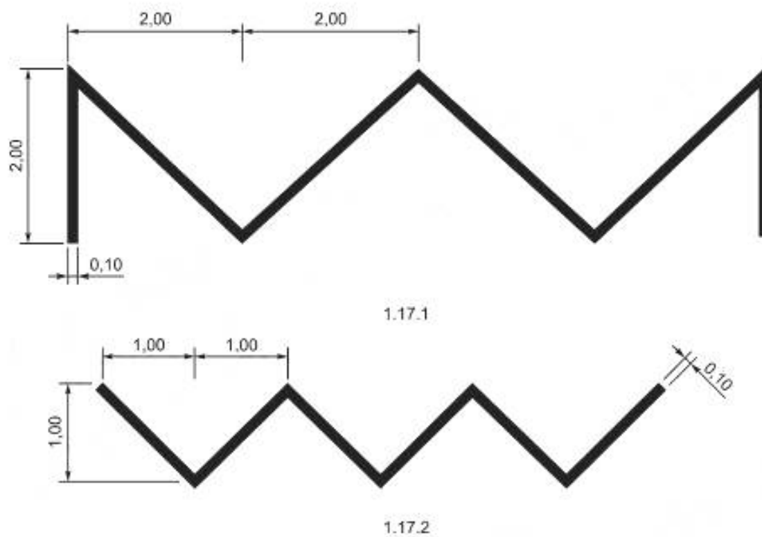
Рисунок Б.4 — Размеры разметки 1.17.1 и 1.17.2
