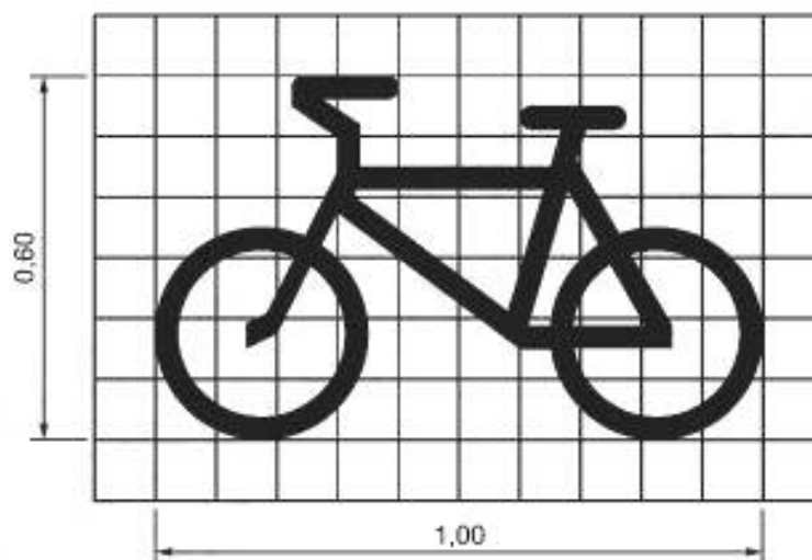
Рисунок Б.13 — Размеры разметки 1.23.3
