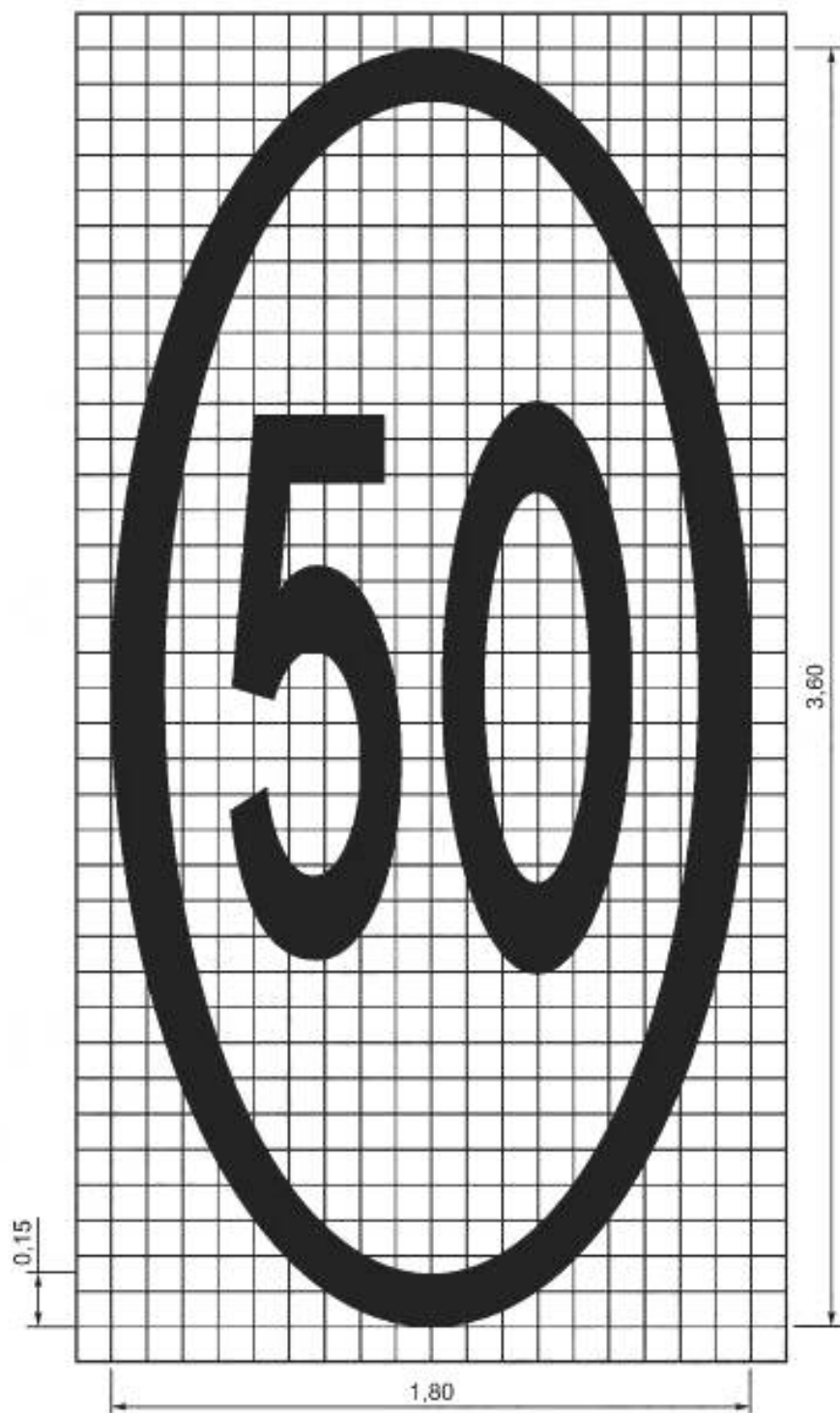
Рисунок Б.15 — Размеры разметки 1.24.2
