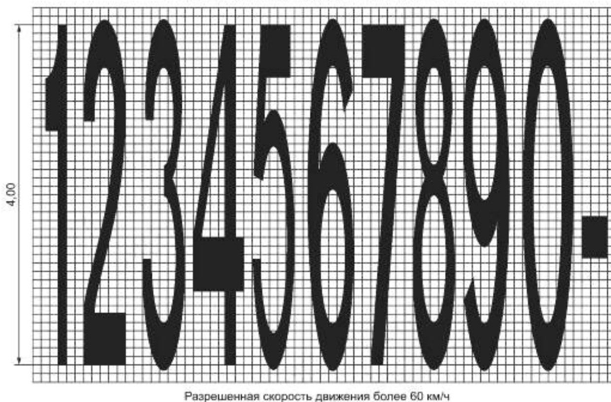
Рисунок Б.9 — Расположение и размеры цифр разметки типа 1.22
