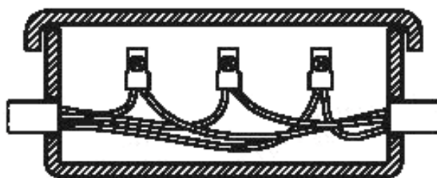
Рисунок АА.1 — Четыре примера соединительных коробок/корпусов
