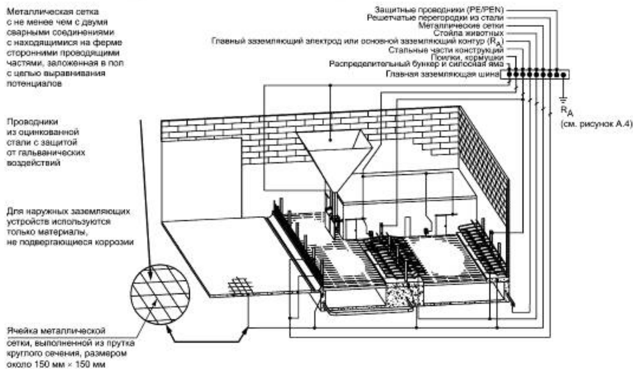
Рисунок А1 — Пример уравнивания потенциалов в коровнике
