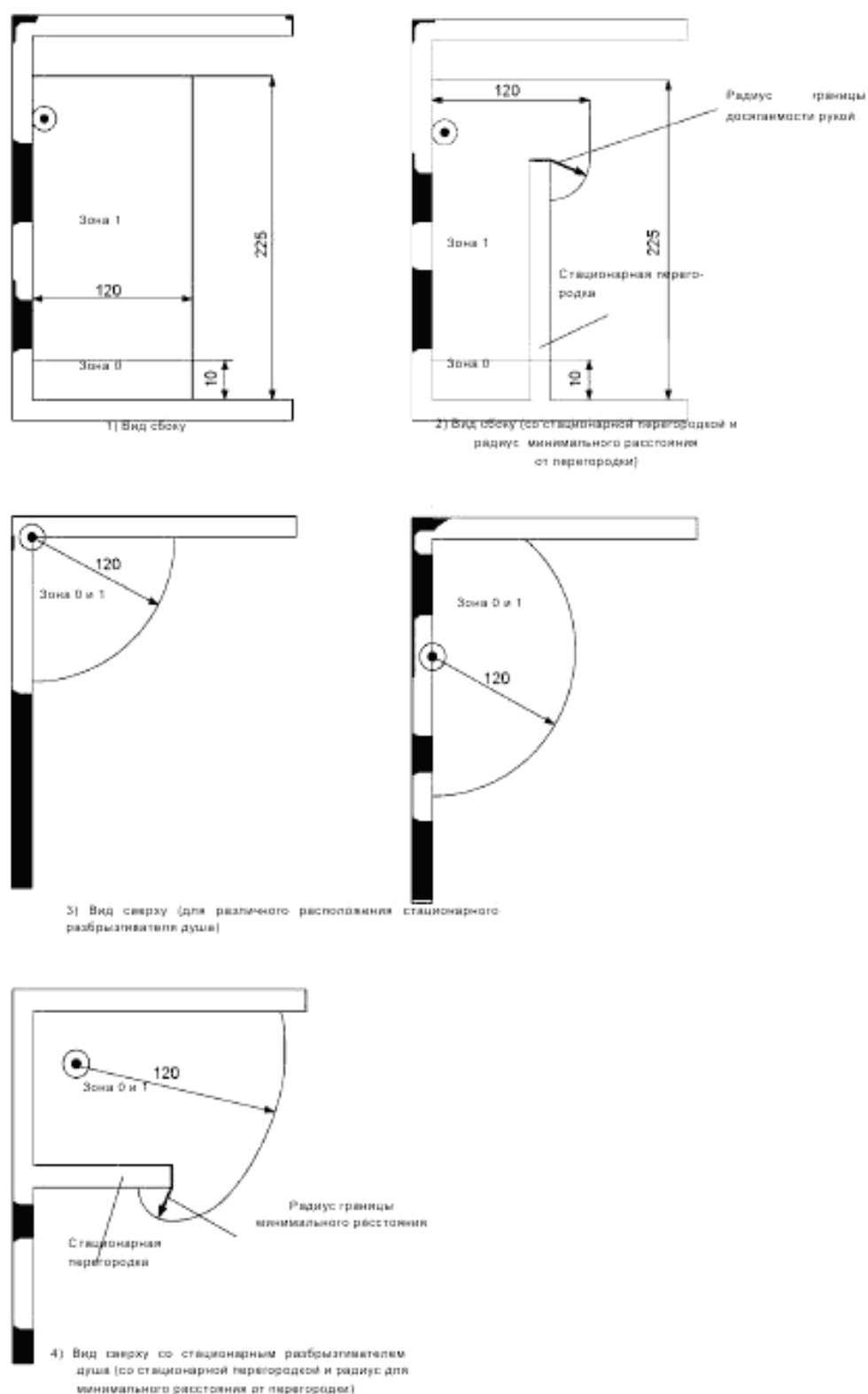
Рисунок 701.2 – Размеры зоны 0 и 1 в помещениях, содержащих душ без поддона
