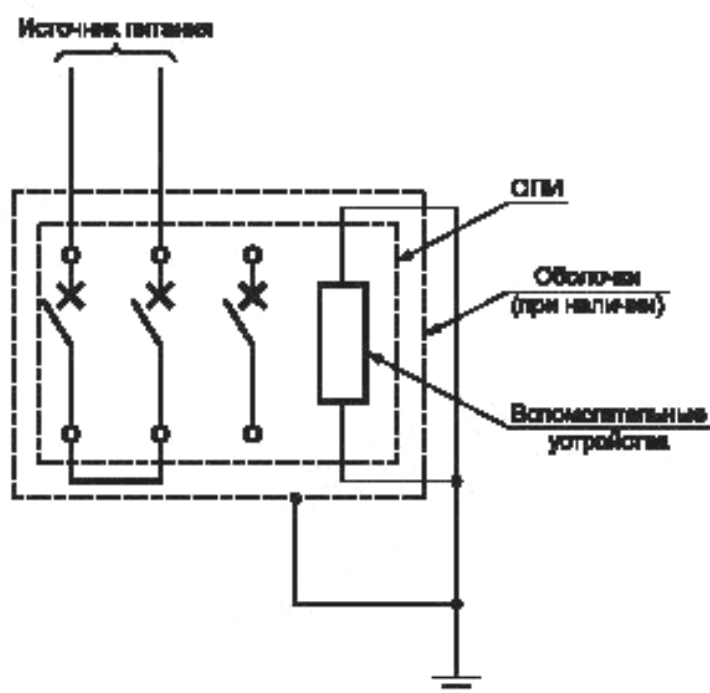
Рисунок F.2 — Испытательная цепь для проверки устойчивости к низкочастотным электромагнитным помехам и испытаний на помехоэмиссию по F.4.1.3, F.4.2, F.4.3, F.4.6, F.4.7.1, F.5.4 и F.6.2 для двух фазных полюсов, соединенных последовательно
