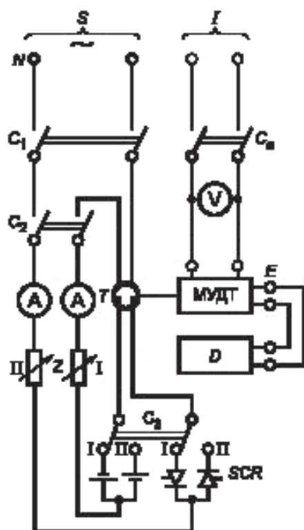
МУДТ с отдельным датчиком
