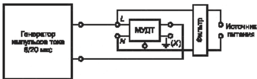
в) МУДТ выводного типа
