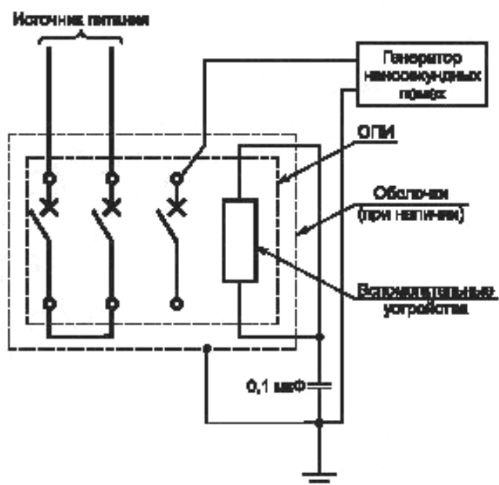
Рисунок F.6 — Цель для проверки устойчивости к наносекундным импульсным помехам по F.4.4 для двух фазных полюсов, соединенных последовательно
