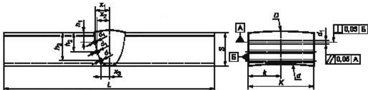
е) НО для УЗК АСС цилиндрических ОК со снятым усилением и расположением БЗО по границе сплавления
