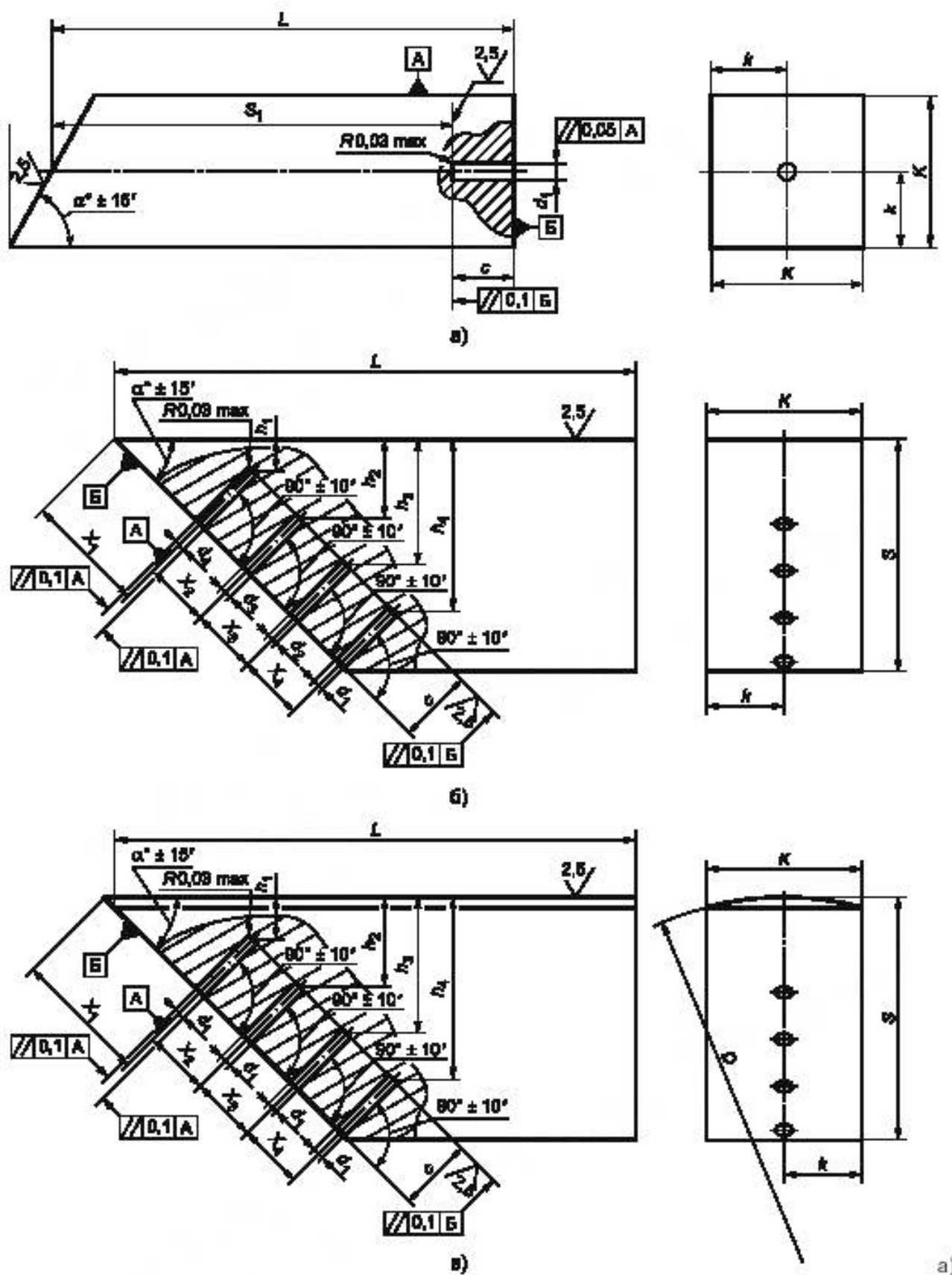
Рисунок 34 — Настройный образец с плоскостными отверстиями для ультразвукового контроля наклонными ультразвуковыми преобразователями
