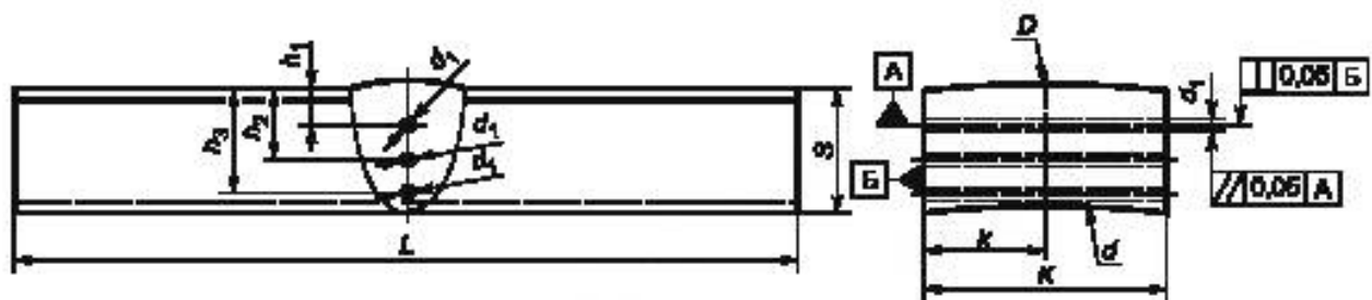
и) НО для УЗК АСС цилиндрических ОК со снятым усиением и расположением БЦО по центру СС
