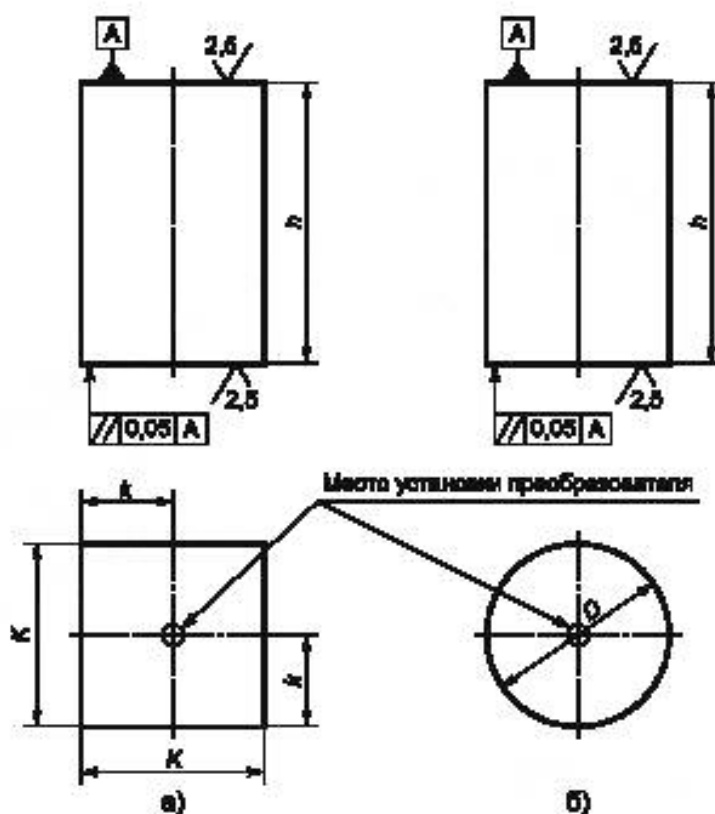
Рисунок 42 — Настройочные образцы для измерения толщины монометаллов (тип T2)
