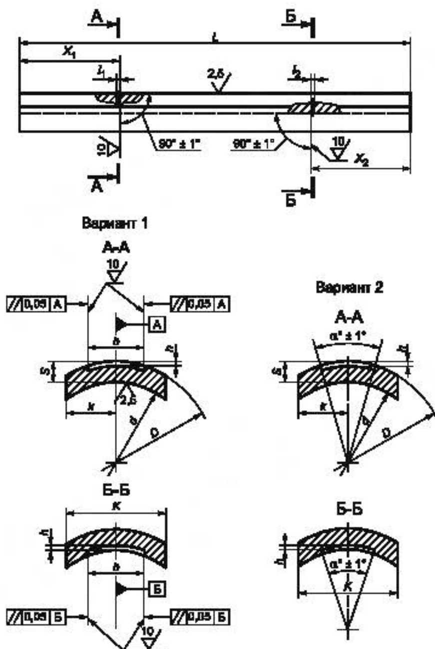
Рисунок 17 — Настрочный образец с протяженными пазами
