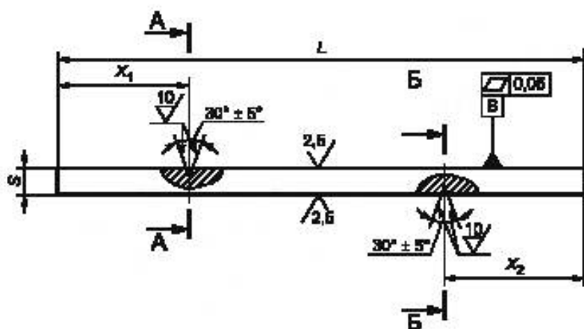
Рисунок 10 — Настроечный образец с зарубками
