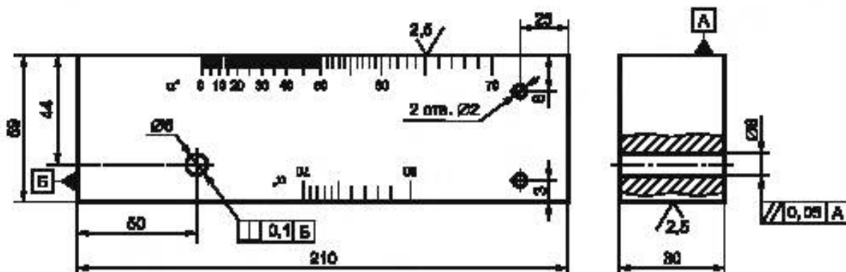
Рисунок 1 — Образец СО-2 (материал — Ст. 20 или Ст. 3)
