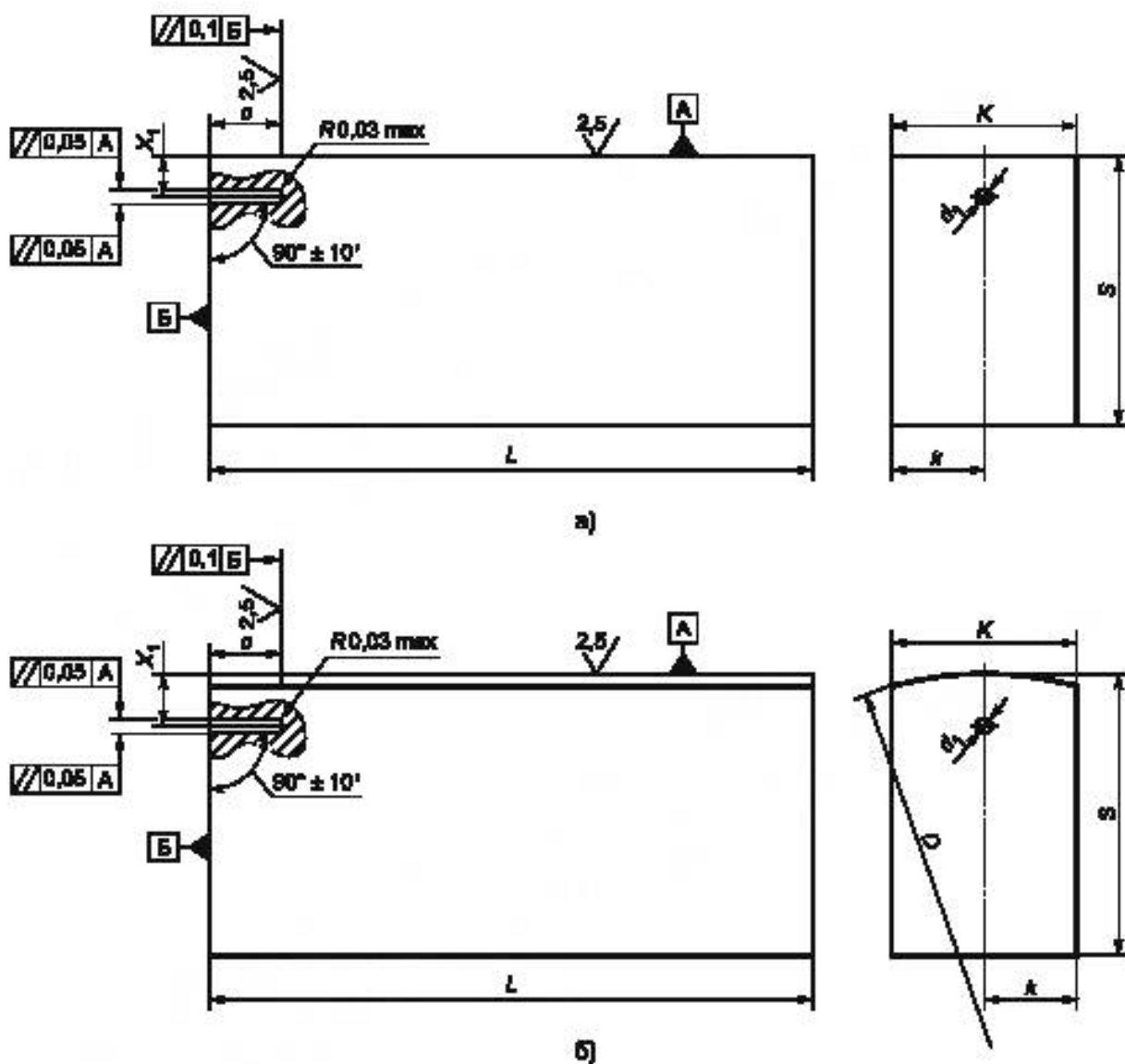
Рисунок 37 — Настройный образец с плоскодонным отверстием для ультразвукового контроля пьезоэлектрическим преобразователем головной волны
