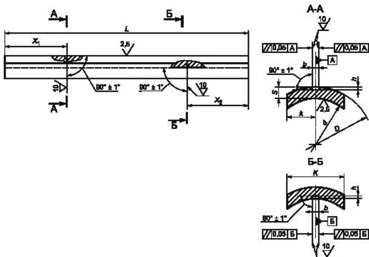
Рисунок 18 — Настроенный образец с зарубками
