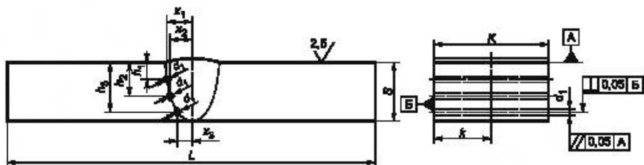
д) НО для УЗК АСС плоскопараллельных ОК со снятым усилением и расположением БЗО по границе сплавления
