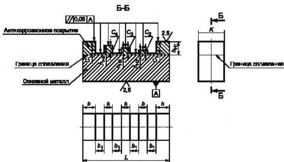
Рисунок 49 — Настроенный образец для измерения толщины антикоррозионного покрытия со стороны основного металла (тип ТН1)
