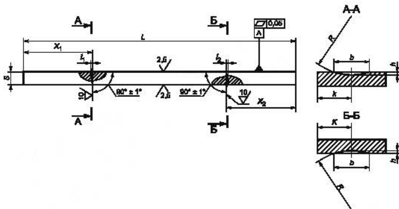
Рисунок 14 — Настроечный образец с сегментными пазами
