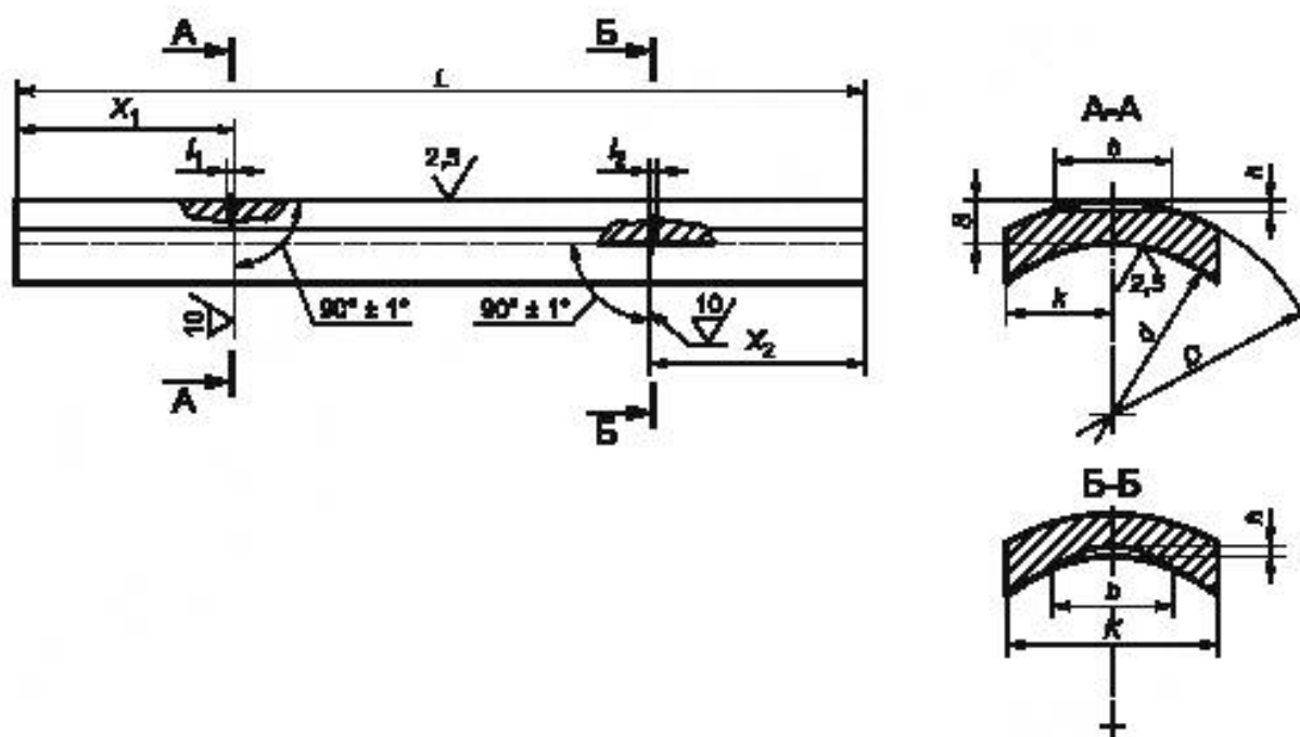
Рисунок 20 — Настроечный образец с сегментными пазами
