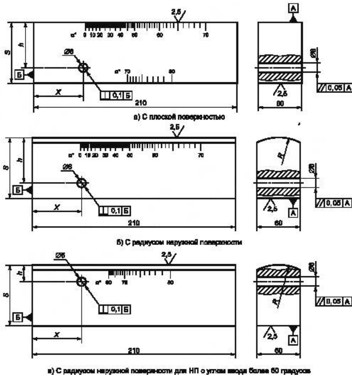
Рисунок 52 — Эскиз НО-СО-2А
