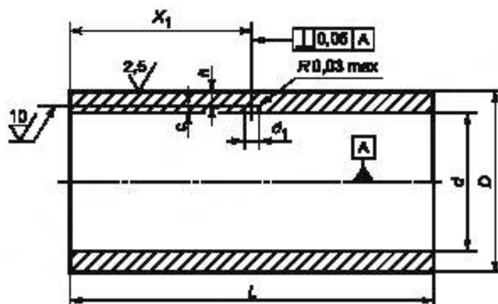
Рисунок 39 — Настроечный образец с плоскодонным отверстием для ультразвукового контроля на расслоение
