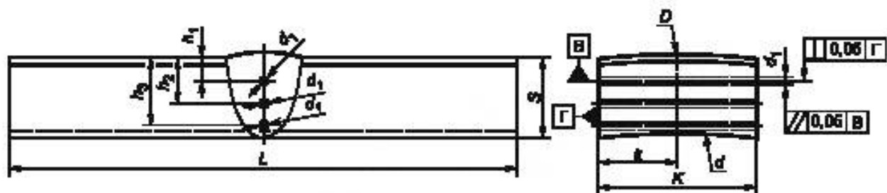
г) НО для УЗК АСС цилиндрических ОК с усилением и расположением БЗО по центру СС
