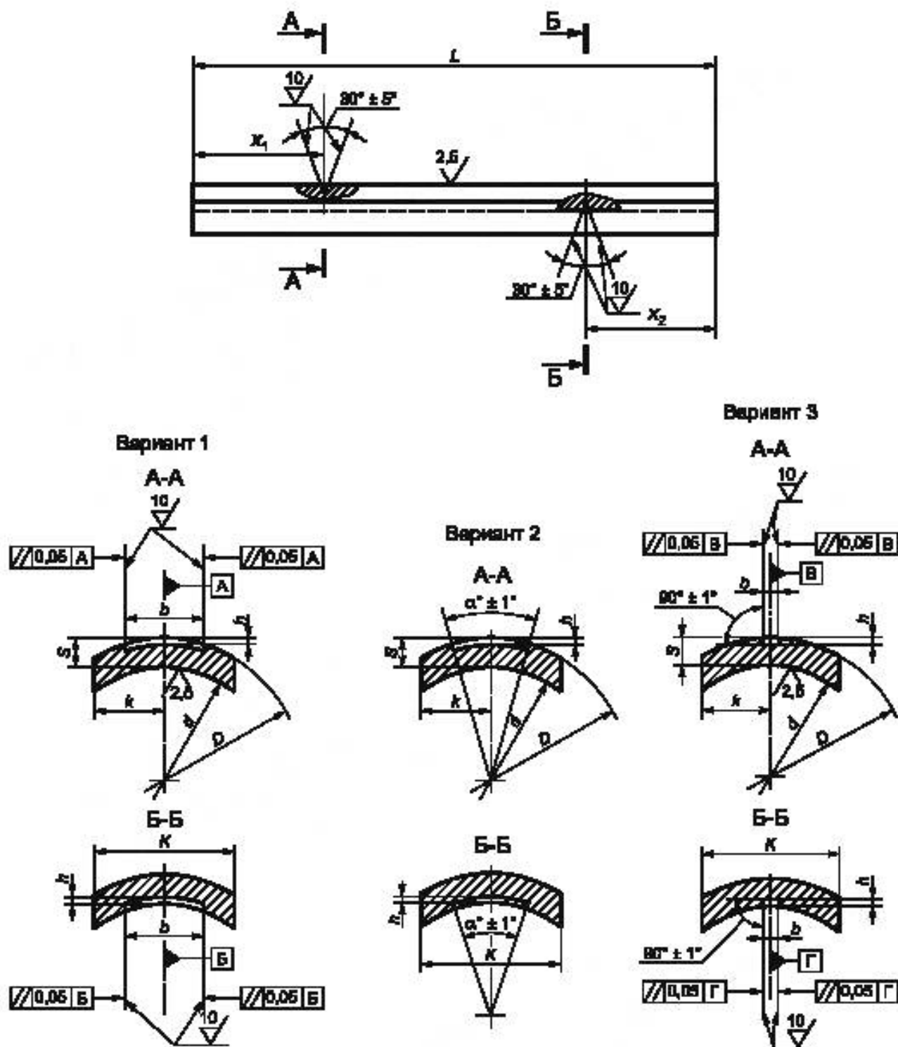
Рисунок 19 — Настроечный образец с рисками
