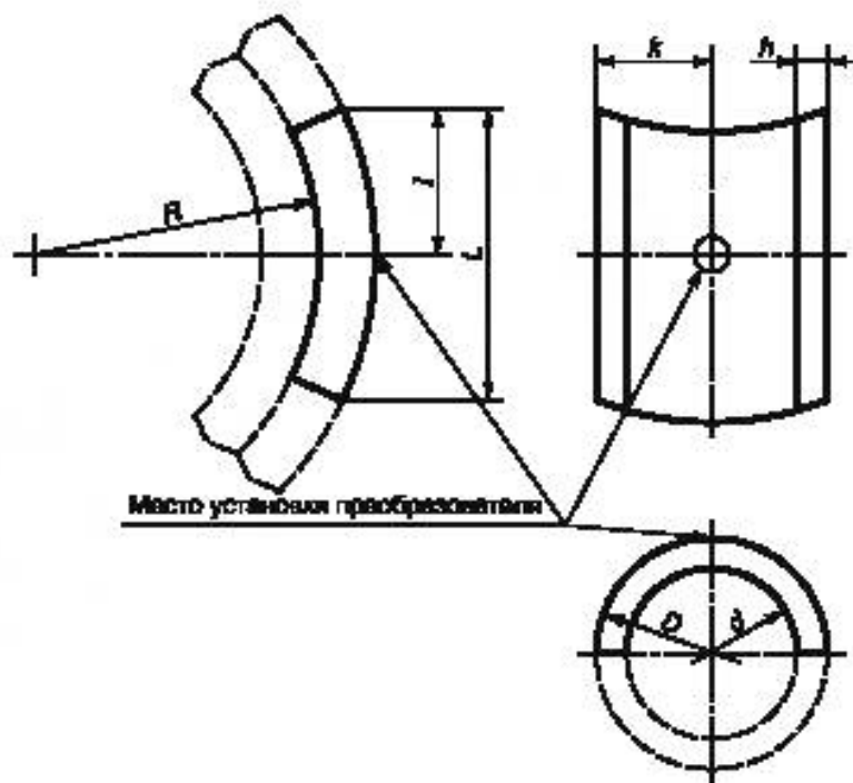
Рисунок 48 — Настроенный образец для измерения толщины гибов
