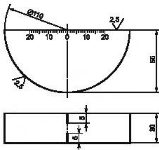
Рисунок 2 — Образец СО-3 (материал — Ст. 20 или Ст. 3)
