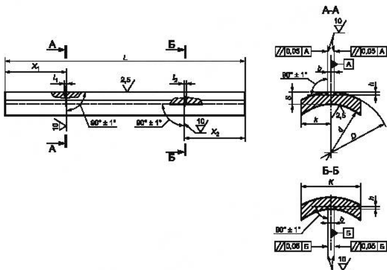
Рисунок 16 — Настроечный образец с пазами
