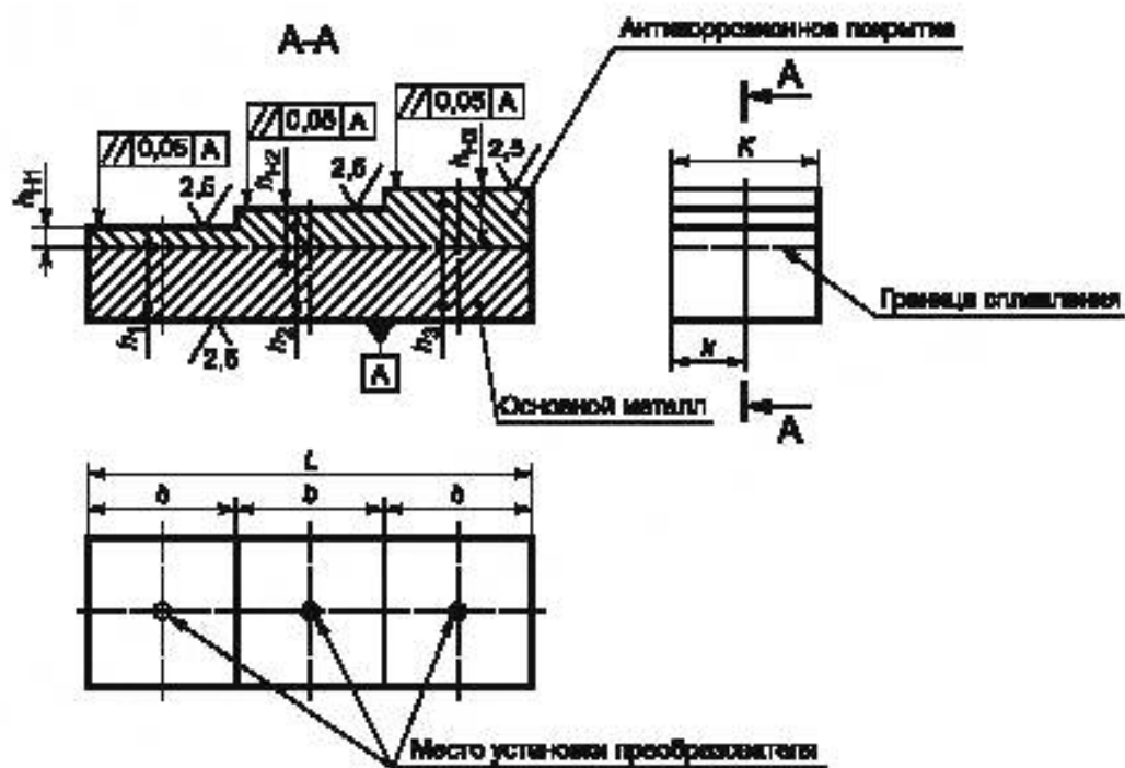
Рисунок 45 — Настроечный образец для измерения толщины биметаллов
