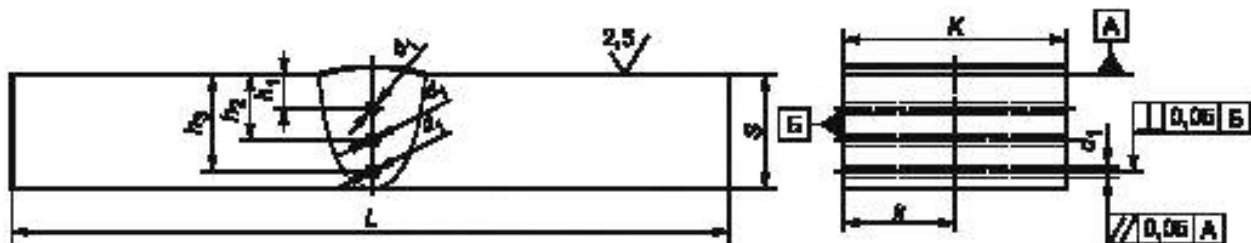
ж) НО для УЗК АСС плоскопараллельных ОК со снятым усилением и расположением БЗО по центру СС
