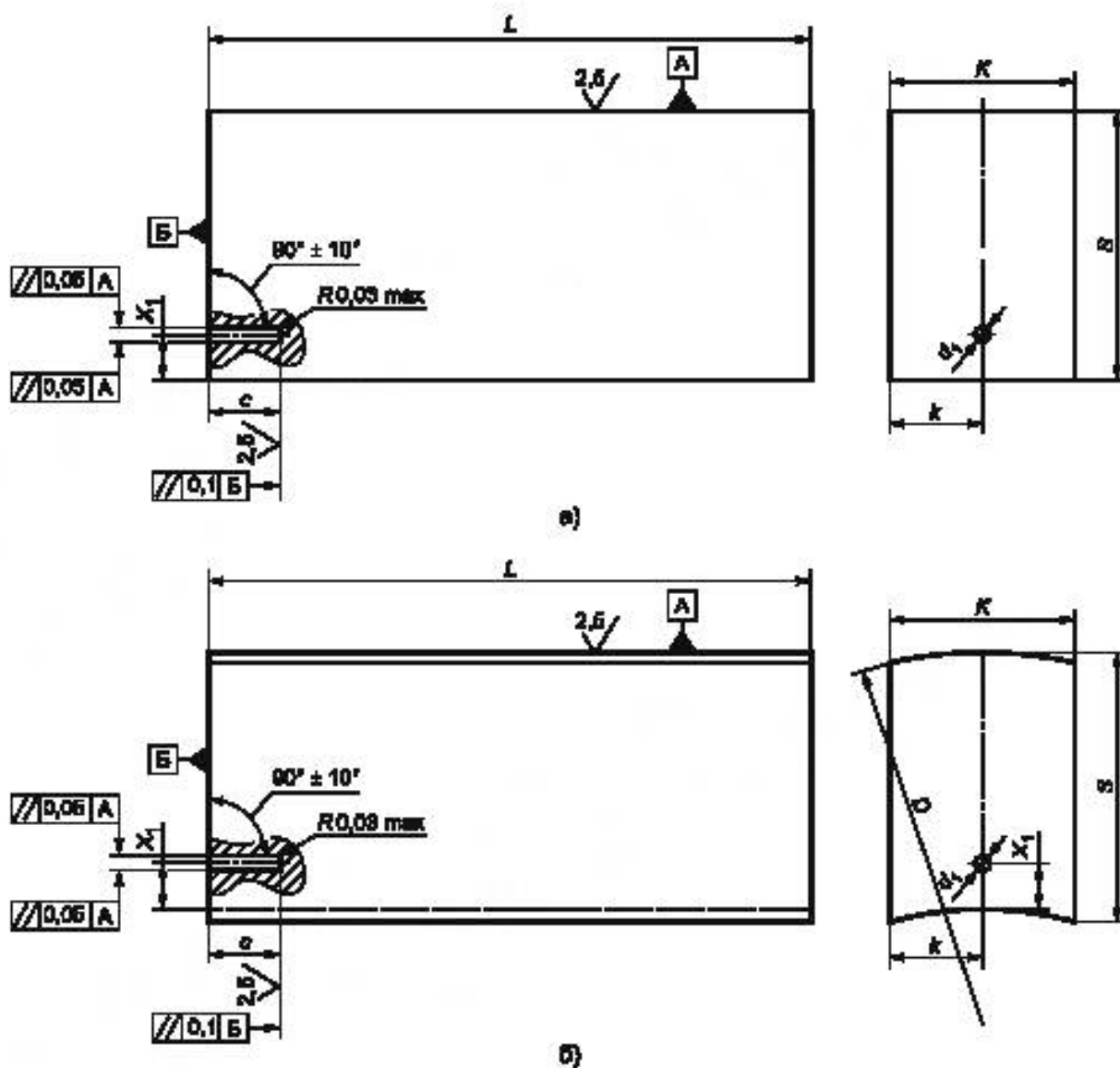
Рисунок 38 — Настроечный образец с плоскодонным отверстием для ультразвукового контроля пьезоэлектрическим преобразователем «корневой тандем»
