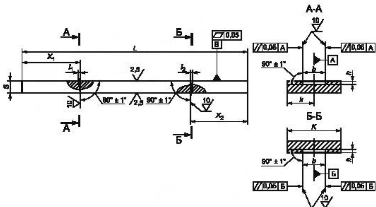
Рисунок 13 — Настроечный образец с протяженными прямоугольными пазами
