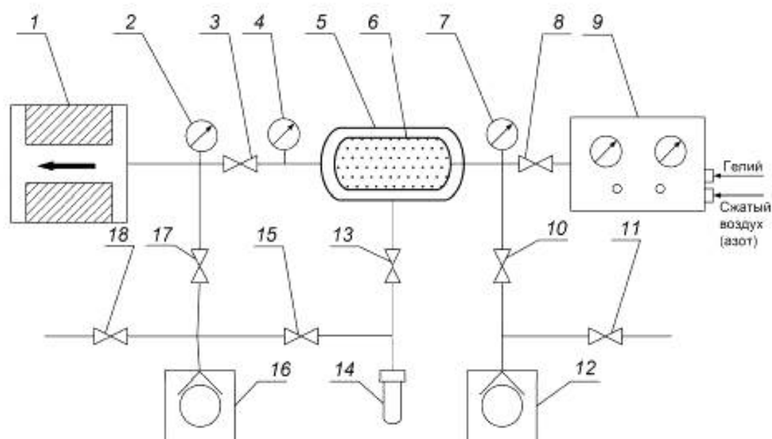
1 — течеискатель; 2, 4 — вакуумметры; 3, 6, 10, 11, 13, 15, 17, 18 — клапаны; 5 — вакуумная камера; 6 — ОК; 7 — мановакуумметр; 9 — пневмолуль; 12, 16 — вакуумные насосы; 14 — контрольная течь
