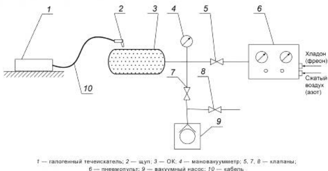
Рисунок 5 — Схема установки для контроля способом галогенного щупа
