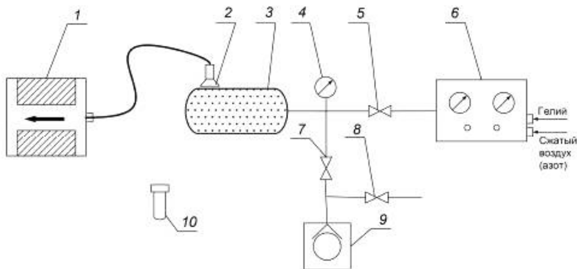
1 — течеискатель; 2 — щуп; 3 — ОК; 4 — мановакуумметр; 5, 7, 8 — клапаны; 6 — пневмоузел; 9 — вакуумный насос; 10 — контрольная течь
