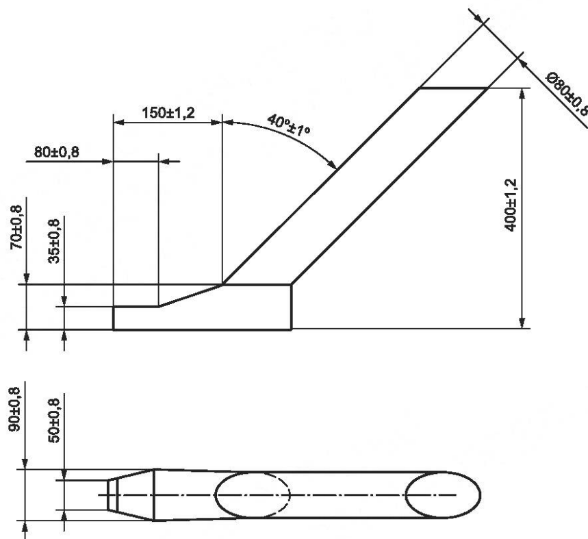
Рисунок 5 — Ножной щуп
