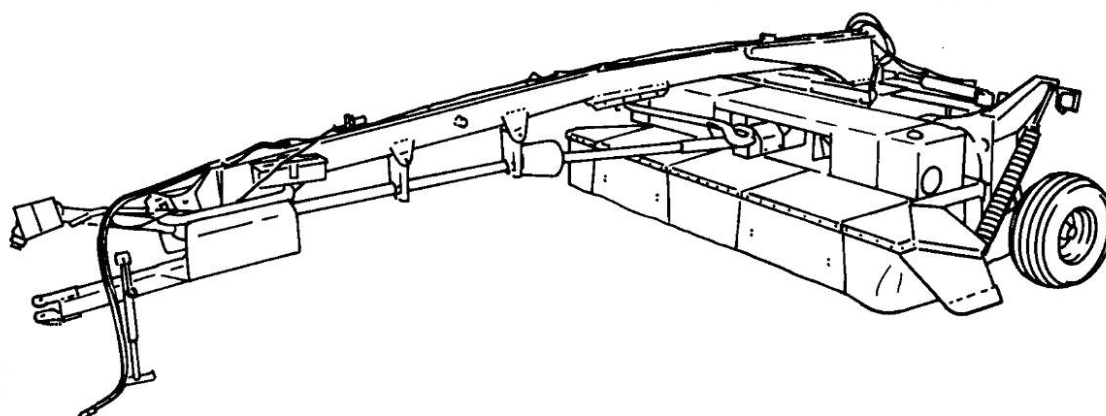
Рисунок А.7 — Ротационная дисковая косилка-плющилка с центральным приводом
