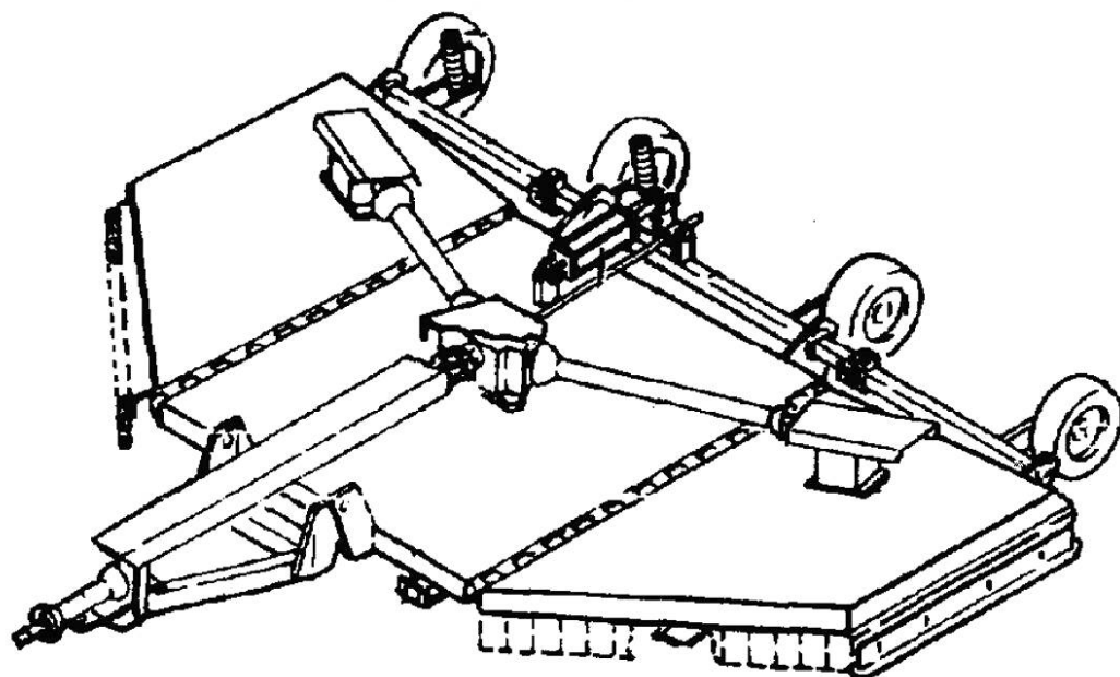
Рисунок А.11 — Многошпиндельная ротационная косилка
