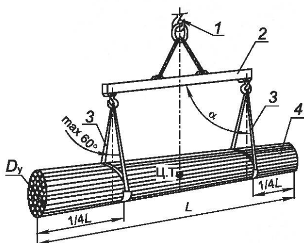
1 — грузозахватный орган подъемного устройства; 2 — грузо-подъемная траверса; 3 — пакетирующий строп; 4 — запакетированный груз; D_y — условный диаметр пакета груза; L — длина пакета груза; \alpha — угол ( 90^\circ \pm 5^\circ )
