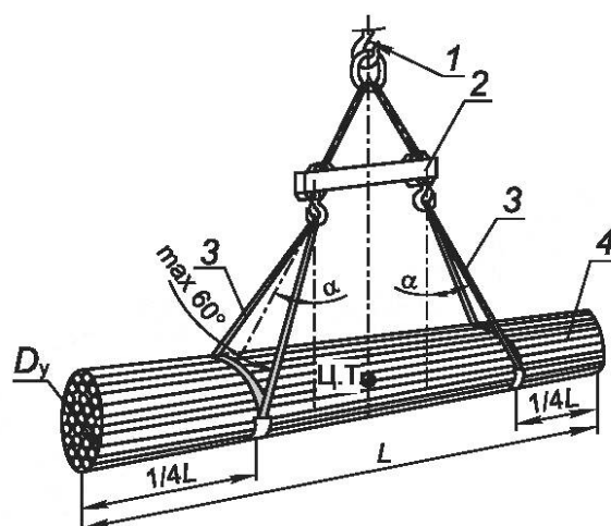
1 — грузозахватный орган подъемного устройства; 2 — грузо-подъемная траверса; 3 — пакетирующий строп; 4 — запакетированный груз; D_y — условный диаметр пакета груза; L — длина пакета груза; \alpha — угол наклона стропов к вертикали (не более 45^\circ )
