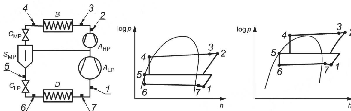
d) Двухступенчатая холодильная установка с отделителем жидкости на ступени промежуточного давления
