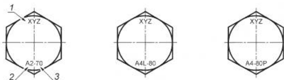
1 — товарный знак изготовителя; 2 — марка стали; 3 — класс прочности
