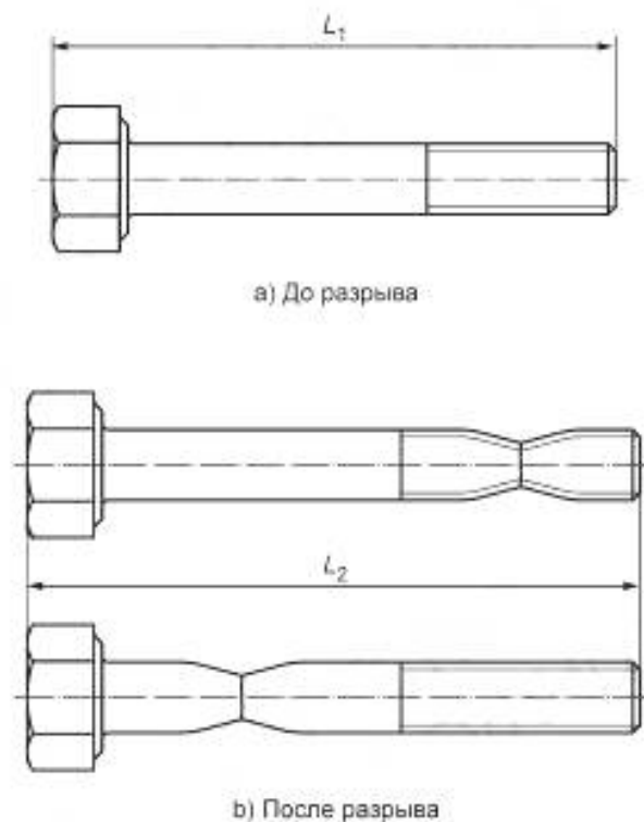
Рисунок 8 — Определение удлинения после разрыва A
