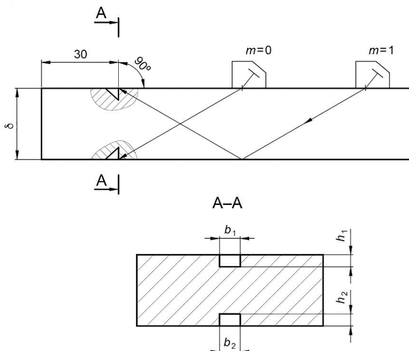
Рисунок А.3 — Эскиз НО с угловыми искусственными отражателями (зарубки) для настройки предельной чувствительности
