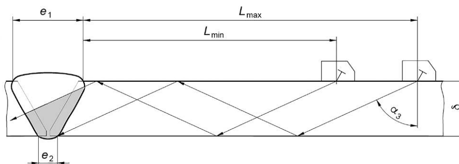
б — одностороннего стыкового СС
