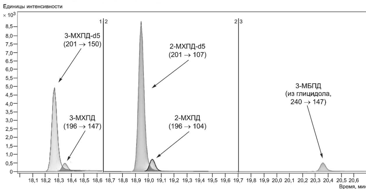
Рисунок Б.1 — Хроматограмма пробы А
