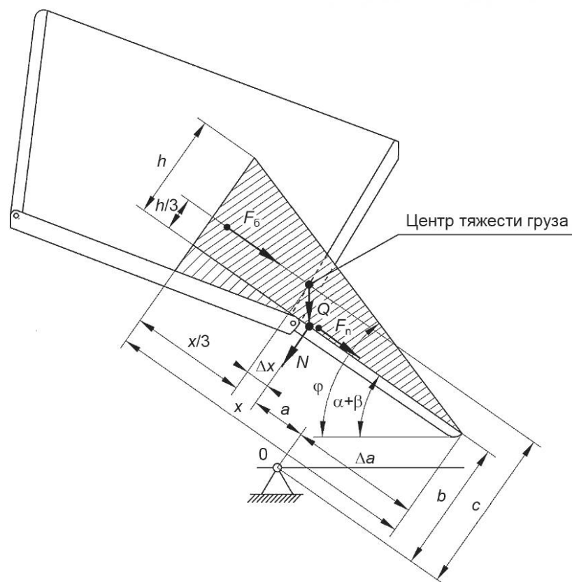
Рисунок A.3 — Схема сил, действующих на кузов вагона от груза (вагон с двусторонней разгрузкой)
