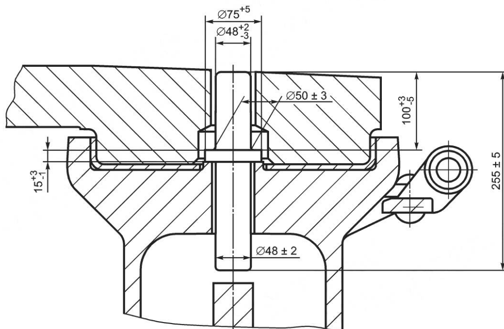
Рисунок Б.1 — Шкворень
