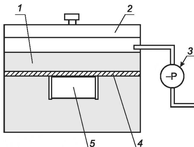
1 — вакуумная камера; 2 — крышка вакуумной камеры; 3 — вакуумметр (манометр); 4 — съемный фиксатор упаковки; 5 — образец упаковки
