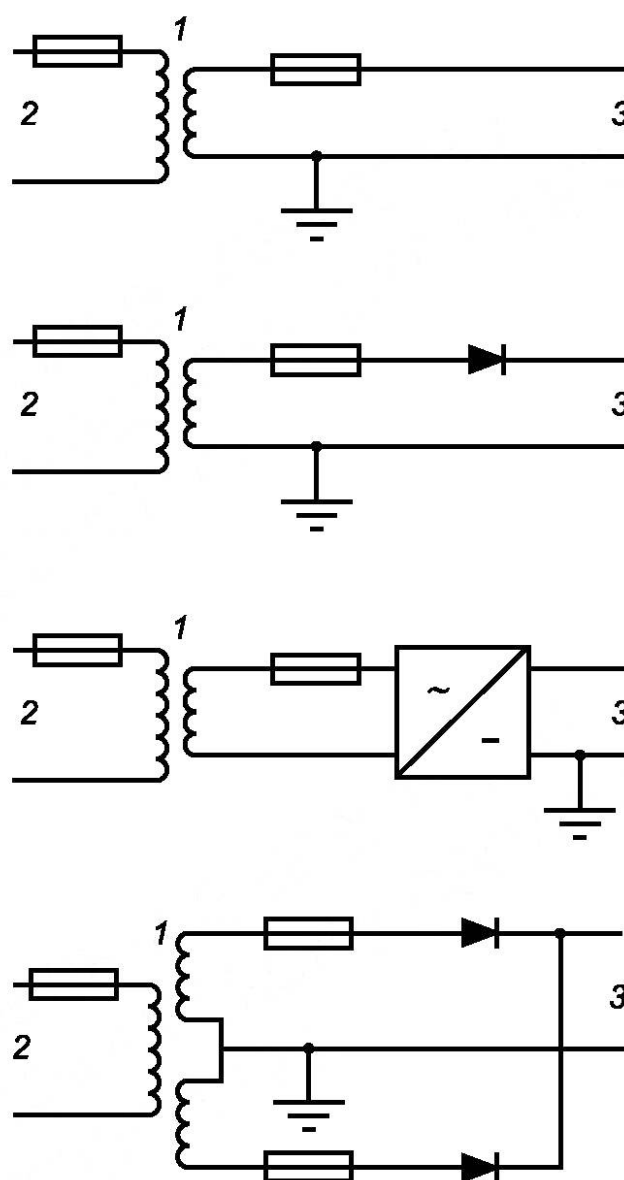
1 — изолирующий трансформатор; 2 — цепь питания; 3 — цепь управления
