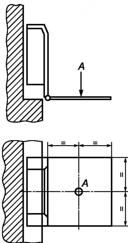
Рисунок 1 — Грузонесущее устройство для пользователя, находящегося в кресле-коляске, или стоящего пользователя
