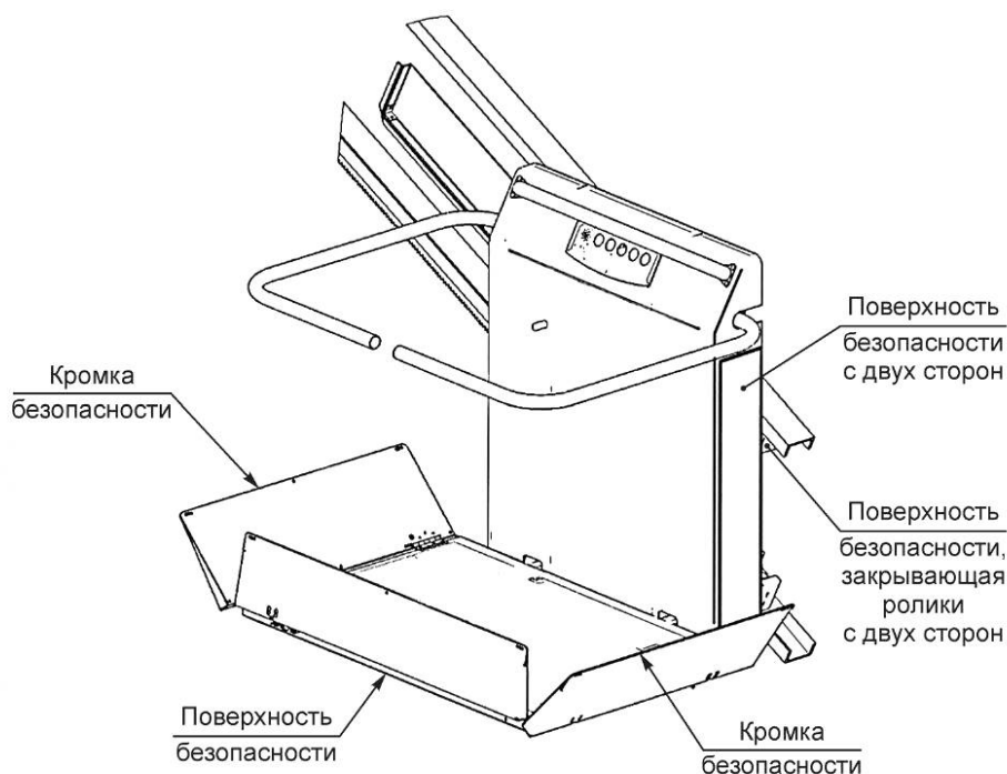
Рисунок 6 — Пример расположения кромок и поверхностей безопасности
