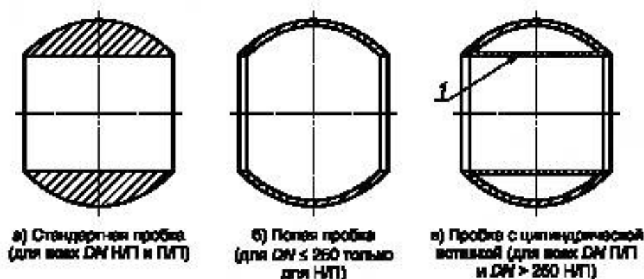
Рисунок 3 — Конструктивные варианты шаровой пробки
