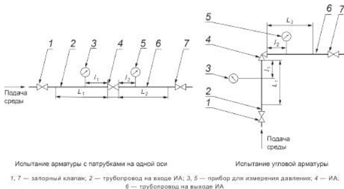
Рисунок 1 — Принципиальная схема испытательного участка гидравлического (пневматического) стенда
