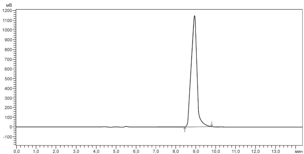
Рисунок А.1 — Образец хроматограммы градуировочного раствора метилового спирта
