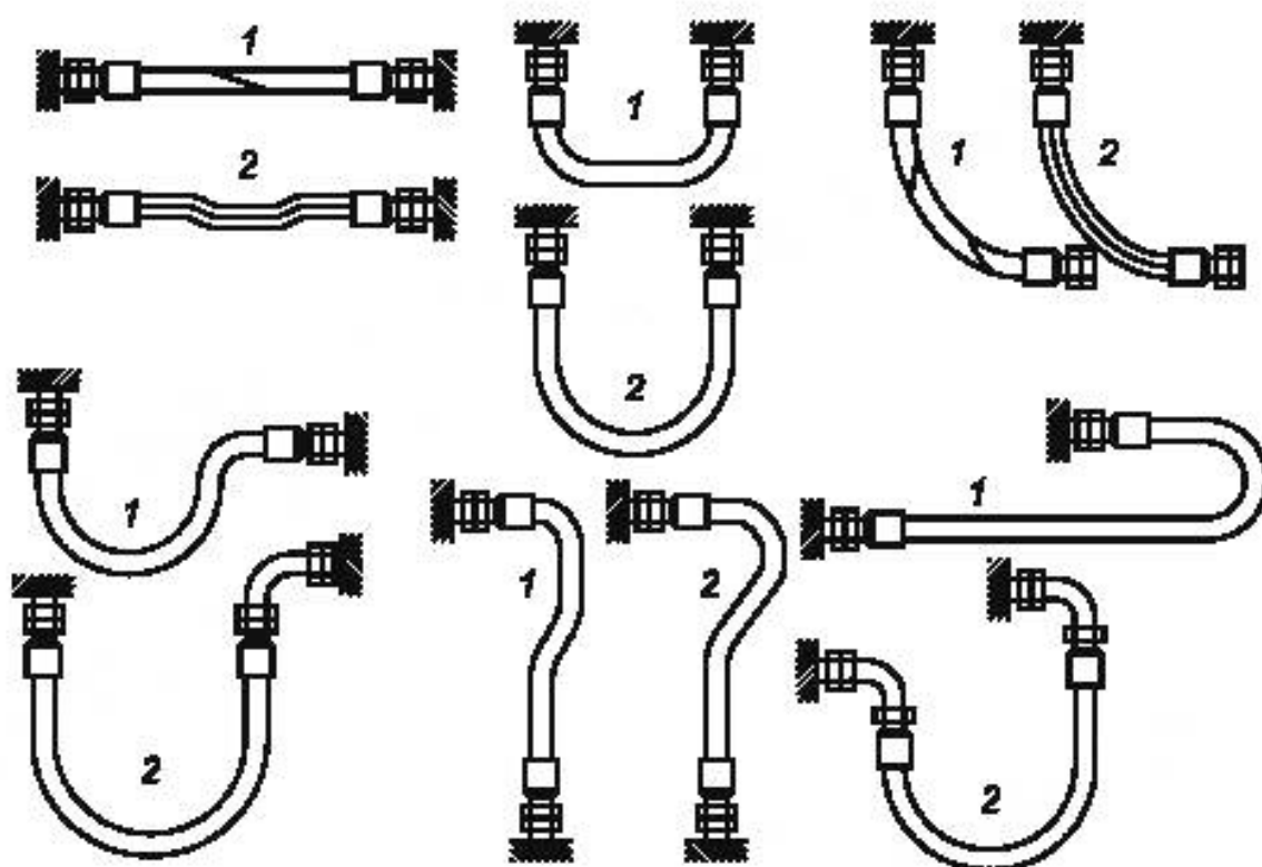
Рисунок 1 — Способы установки гибкого трубопровода: 1 — неправильно; 2 — правильно
