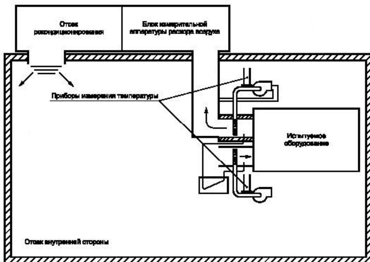
Рисунок F.4 — Компоновка оборудования испытательной камеры для проведения испытаний методом комнаты
