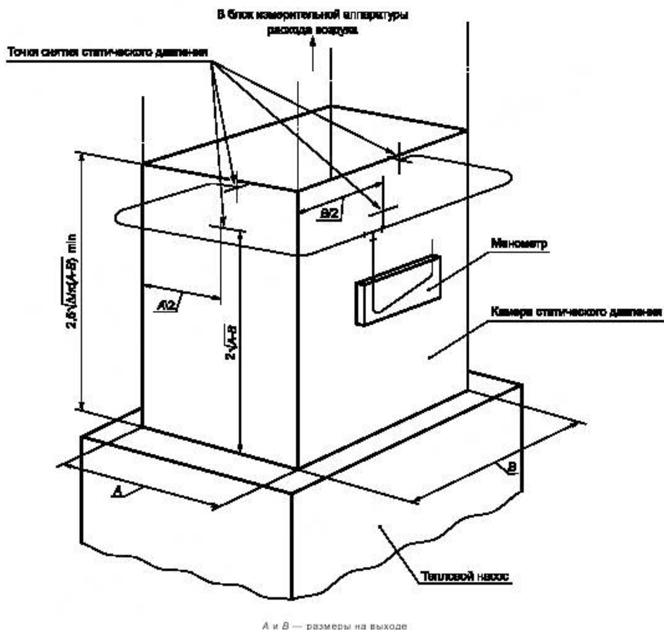
Рисунок F.7 — Измерение внешнего статического давления
