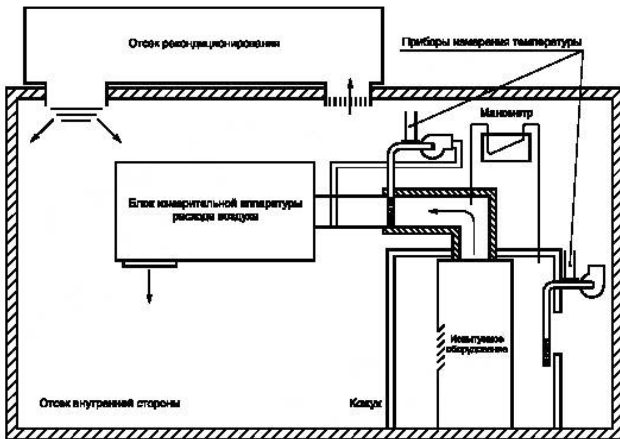
Рисунок F.3 — Компонентное оборудование испытательной камеры для проведения испытаний с использованием кожуха
