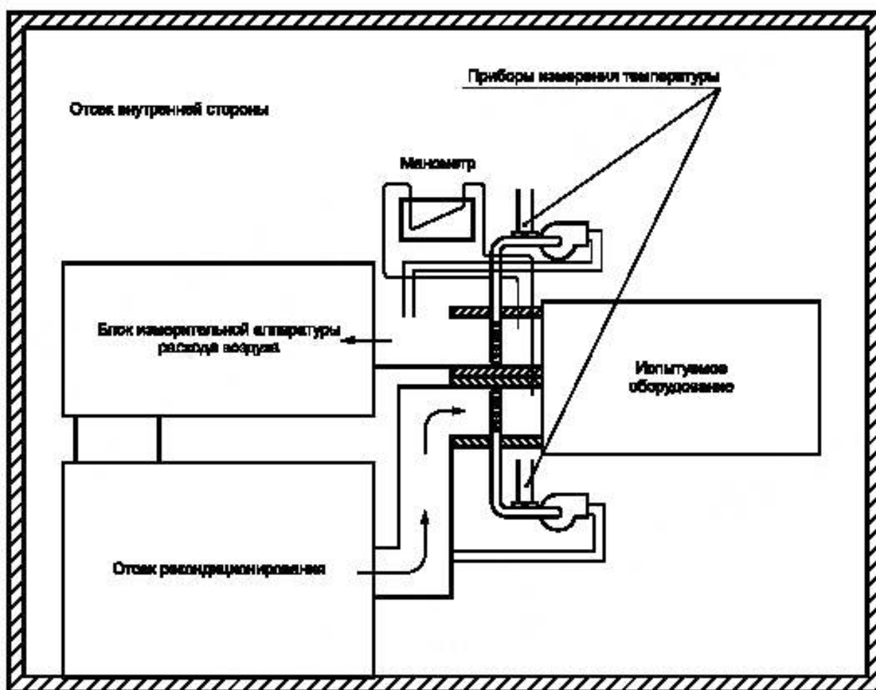
Рисунок F.2 — Компонировка оборудования испытательной камеры для проведения испытаний методом петли
