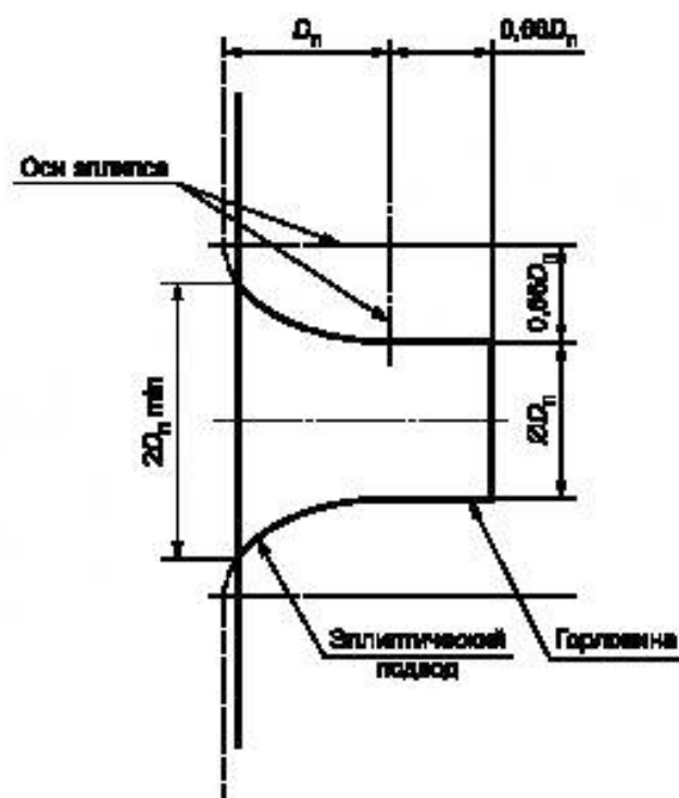
Рисунок F.6 — Сопло для измерения расхода воздуха
