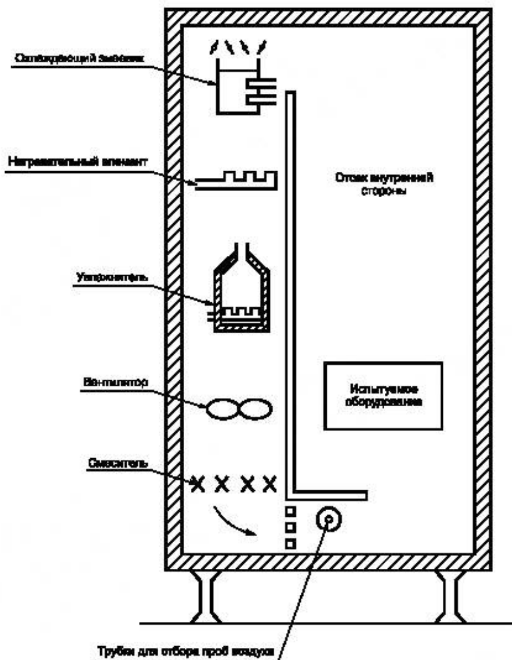
Рисунок Е.1 — Типичный калиброванный калориметр комнатного типа
