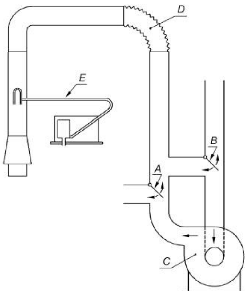
А и В — перегородки для получения восходящей и обратной тяги; С — вентилятор; D — гибкий патрубок; Е — трубка Пито для измерения скорости потока
