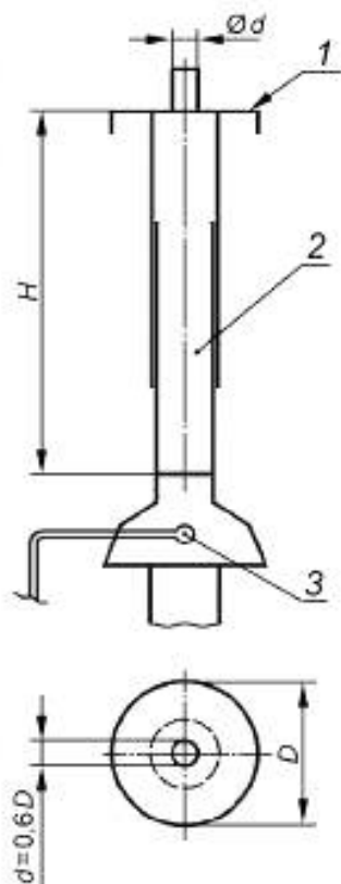
1 — пластина; 2 — телескопический испытательный дымоход; 3 — детектор
