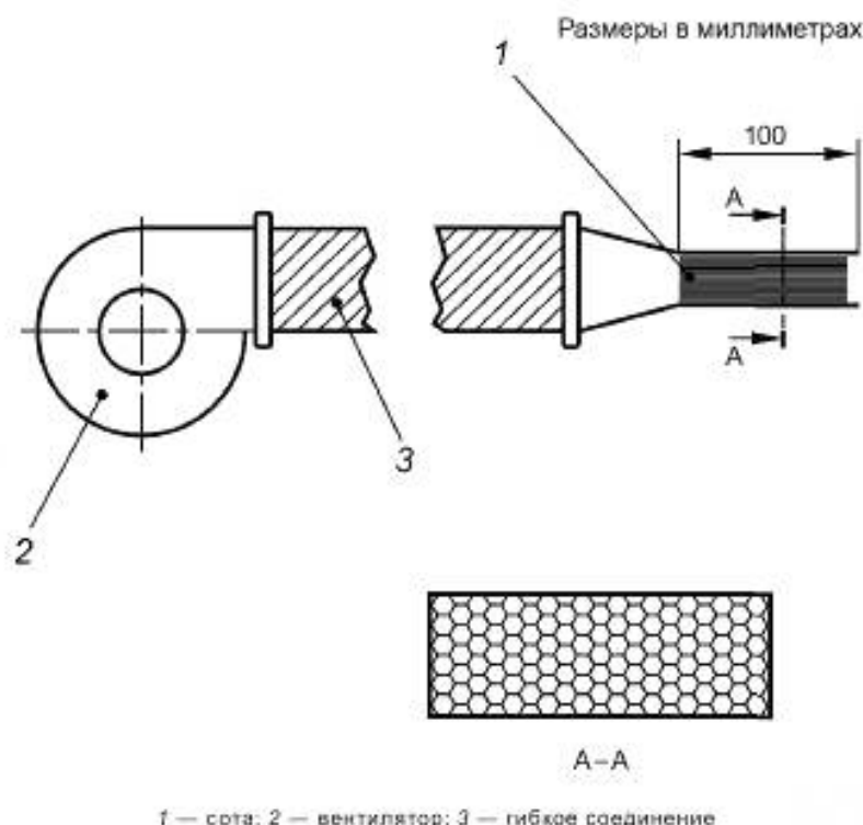
Рисунок 2 — Устройство для испытания на ветровую нагрузку
