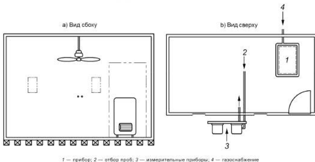
Рисунок F.1 — Пример климатической камеры
