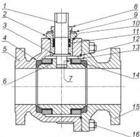
1 — шпindelь; 2 — крышка; 3 — упорное кольцо; 4 — седло; 5 — корпус крана; 6 — шаровая пробка; 7 — радиальный подшипник опоры (подшипник скольжения); 8 — втулка сальника; 9 — крепеж крышки; 10 — уплотнение крышки; 11 — уплотнение шпindеля (сальниковая набивка); 12 — уплотнение корпуса; 13 — плоская опора; 14 — торцевой подшипник опоры (подшипник скольжения); 15 — фланец; 16 — крепеж корпуса
