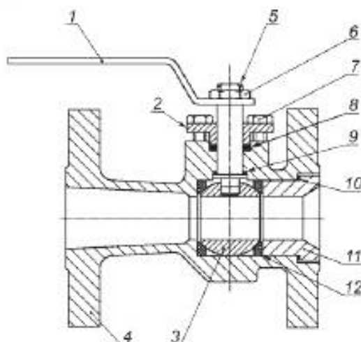
1 — рукоятка; 2 — втулка сальника; 3 — шаровая пробка; 4 — корпус; 5 — шпindelь; 6 — гайка; 7 — крепеж втулки сальника; 8 — сальник; 9 — упорное кольцо; 10 — уплотнение корпуса; 11 — корпусная втулка; 12 — седло
