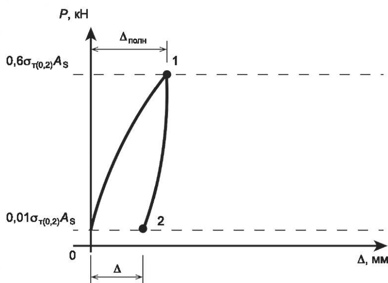
Рисунок 4 — Схема нагружения образцов для определения деформативности первым и вторым способами
