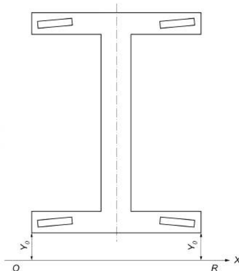
Рисунок 1 — Выбор базовой линии
