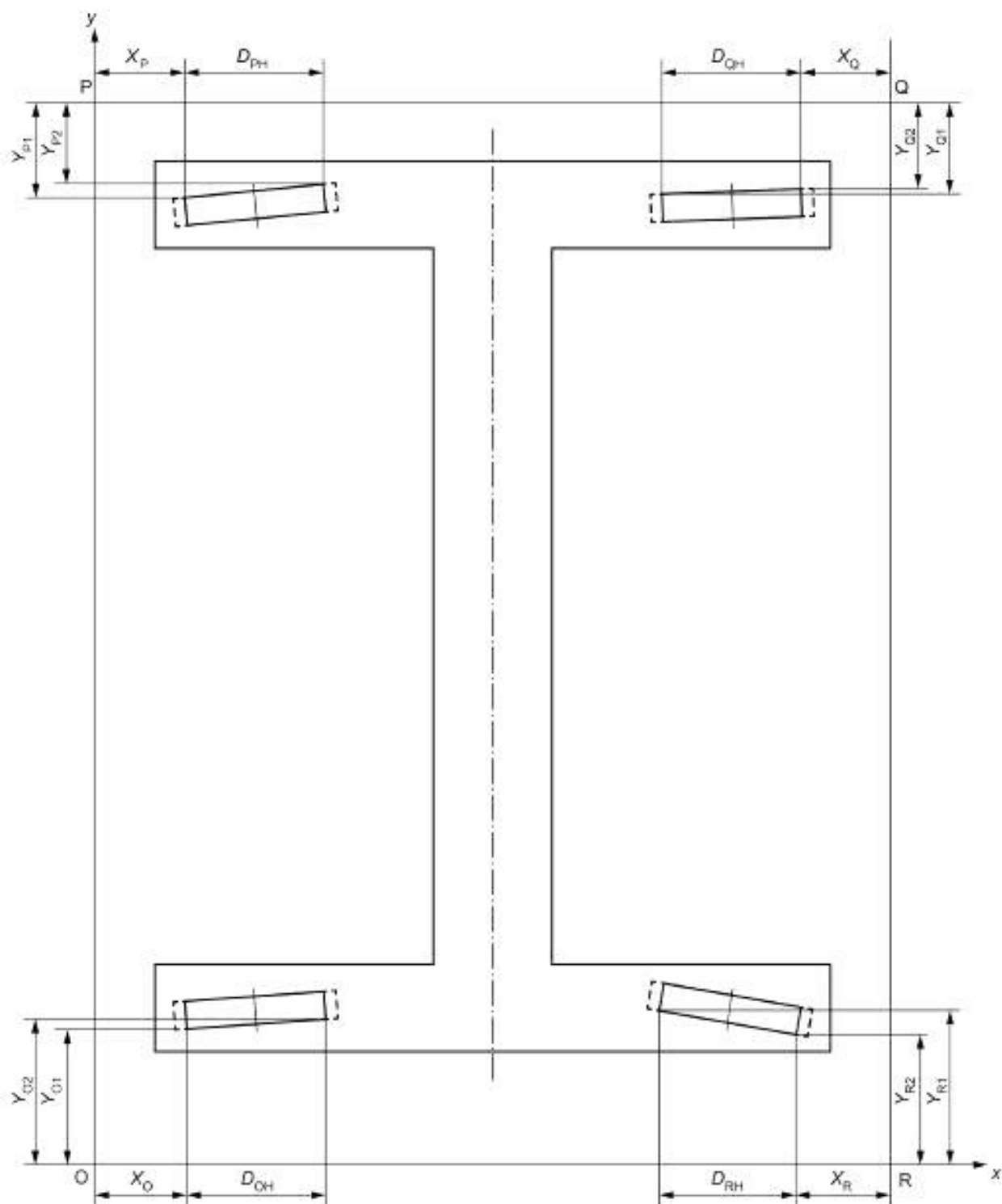
Рисунок 2 — Геодезический прямоугольник и измерения размеров
