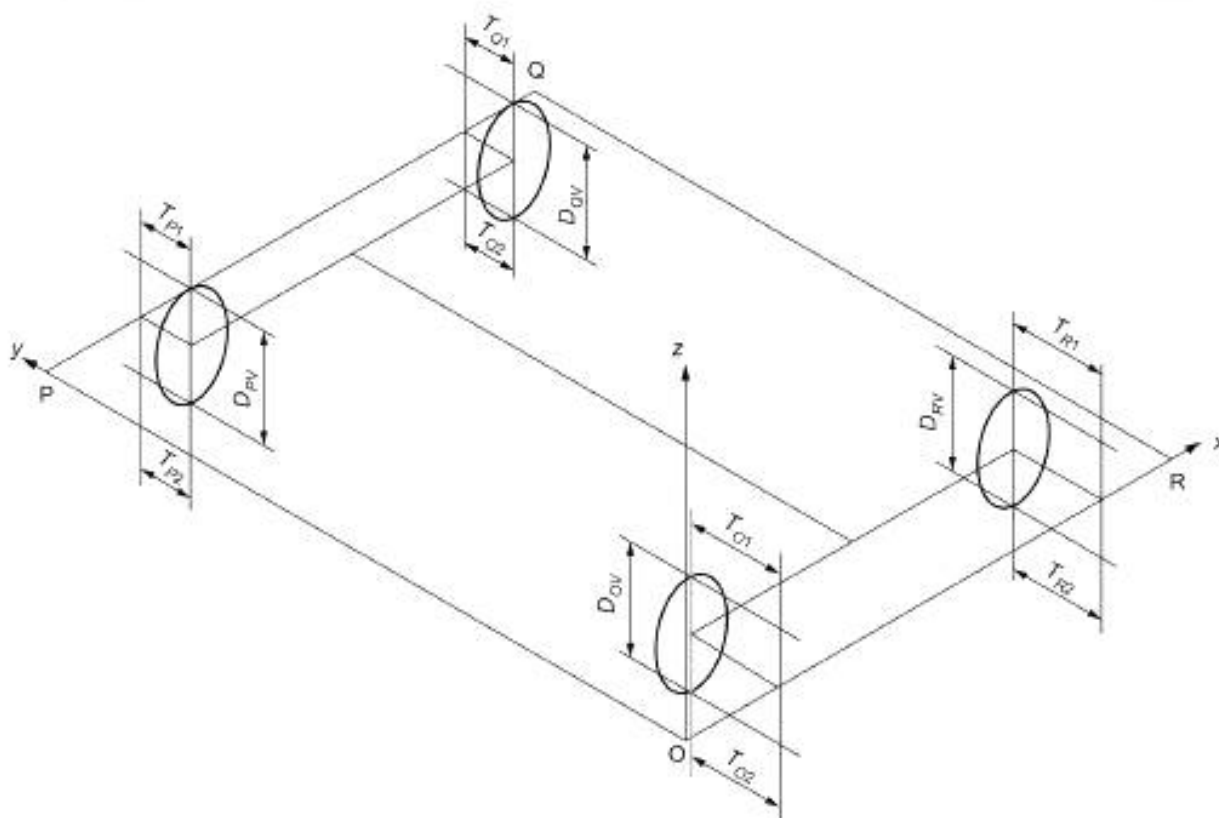
Рисунок 3 — Измерения отклонений положения колес от вертикальной плоскости
